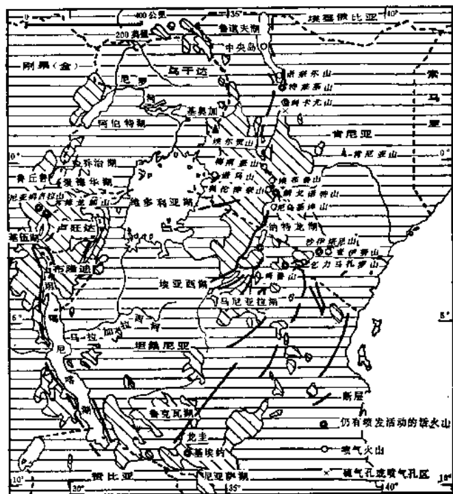
图 164 活火山与主要断层线
