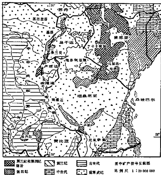
图 163 东非地质略图
