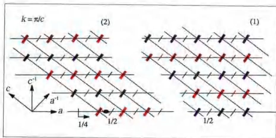
彩图 6.27 Au(1)和Ba(2)的超分子轨道 k=0 和 k=\pi/c 在 (a, c) 平面的示意图 (沿着 c^{-1} 的方向)
