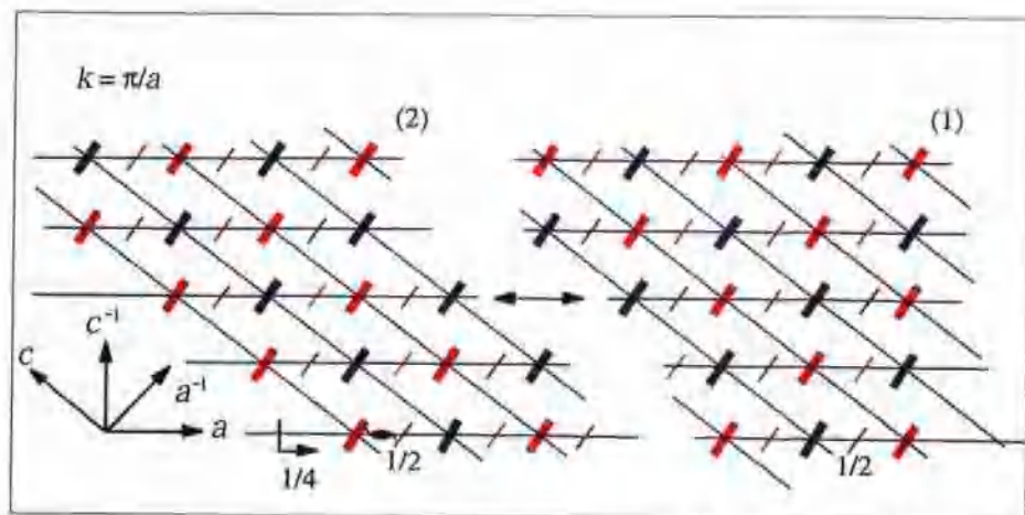
彩图 6.26 Au(1)和Ba(2)的超分子轨道 k=0 和 k=\pi/a 在 (a, c) 平面的示意图 (沿着 a^{-1} 的方向)
