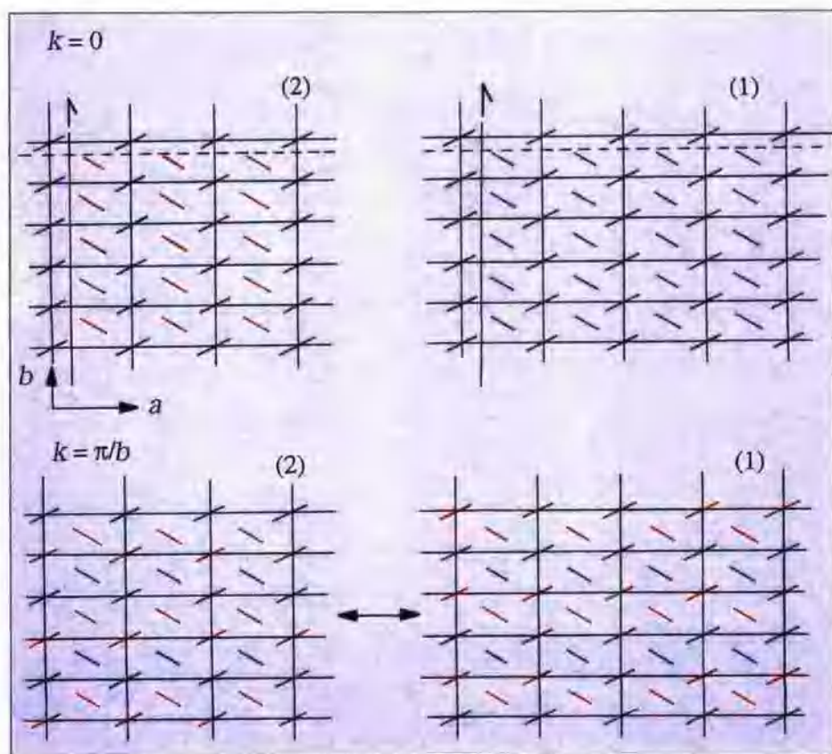
彩图 6.25 Au(1)和Bu(2)的超分子轨道 k=0 和 k=\pi/b 在 (a, b) 平面的示意图(沿着 b^{-1} 的方向), 通常Au具有 2i 的蓝—蓝转换, Bu具有 2i 的蓝—红转换
