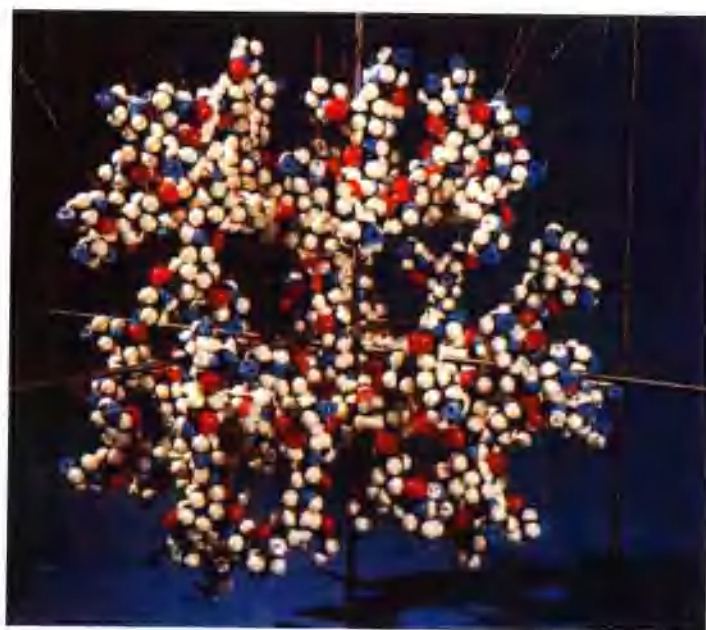
彩图 3.69 PAMAM(Polyamidoamine)树枝状化合物的化学式及其相应的分子模型 (得到了文献[35]中Wiley-VCH的复制许可)
