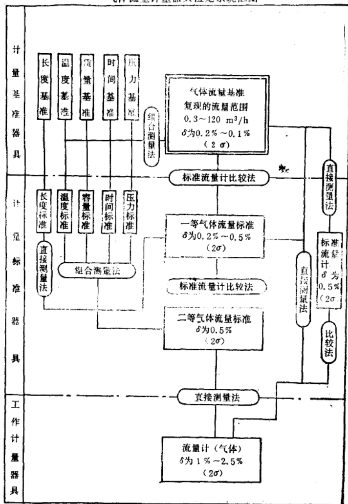
气体流量计量器具检定系统图
