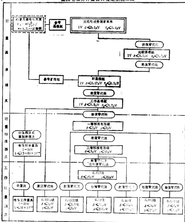
直流电动势计量器具检定系统框图
