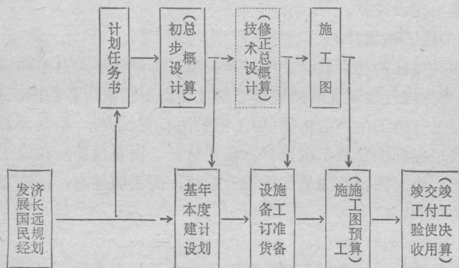
图 1-1 基本建设程序示意图
