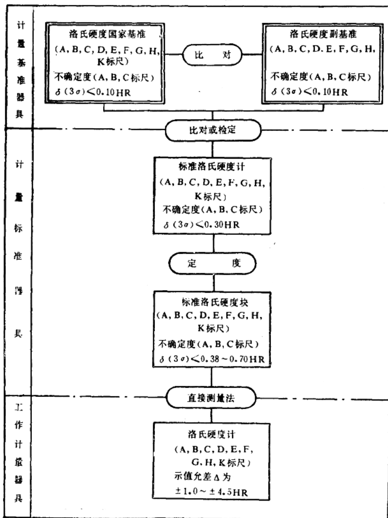
金属洛氏硬度计量器具检定系统框图
