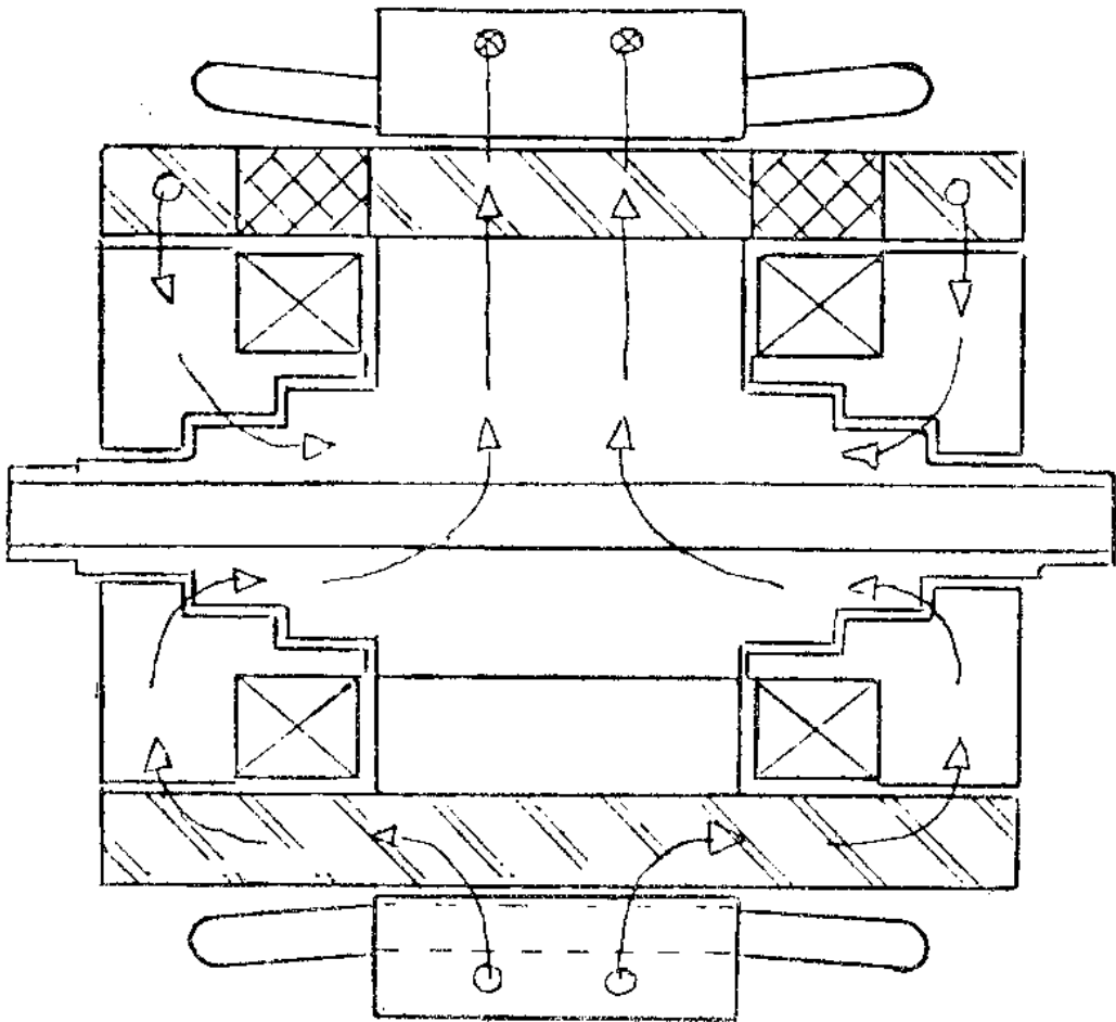
图1.1.1.3A 内线圈、固定式、双线圈伦台尔交流发电机（贝基、罗宾逊） 无刷固定线圈式伦台尔型发电机，使用两个激磁线圈，美国专利2796542所述，A. 贝基发行。
