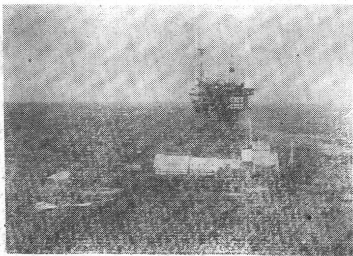
英国北海福蒂斯油田的一座平台
