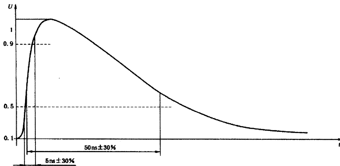
图3 50 Ω 负载时单脉冲波形
