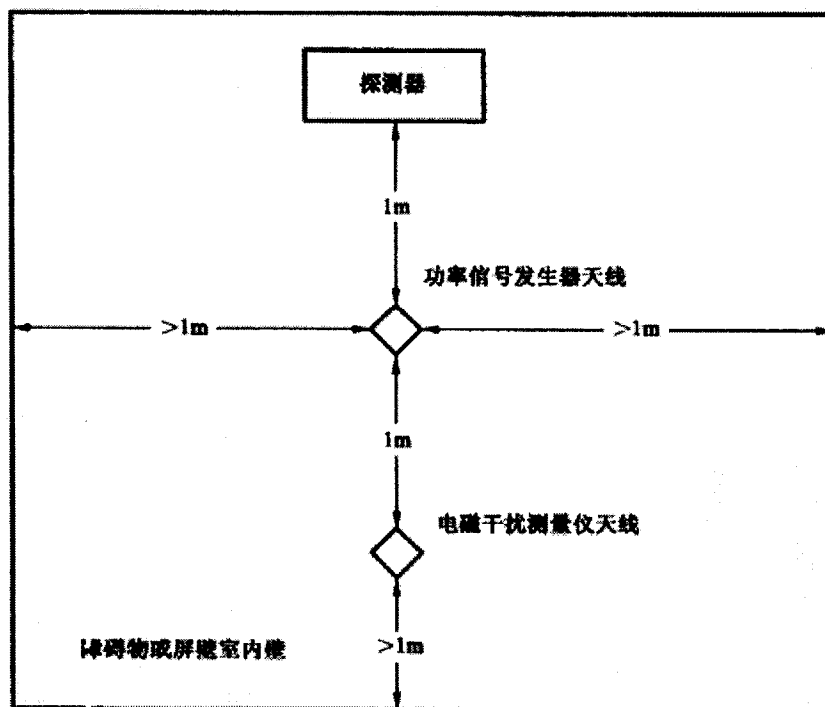
图 2 天线位置图
