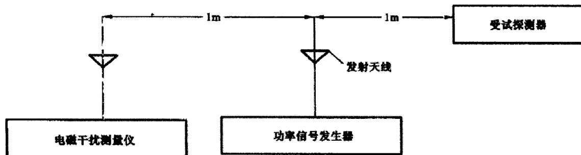
图 1 试验设备布置图
