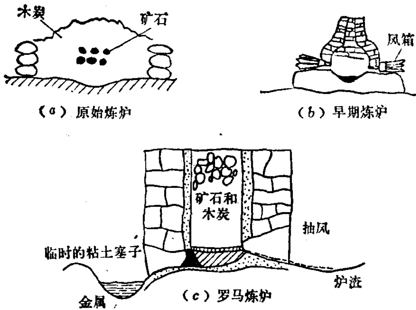
图 1-2 各型古代炼炉
