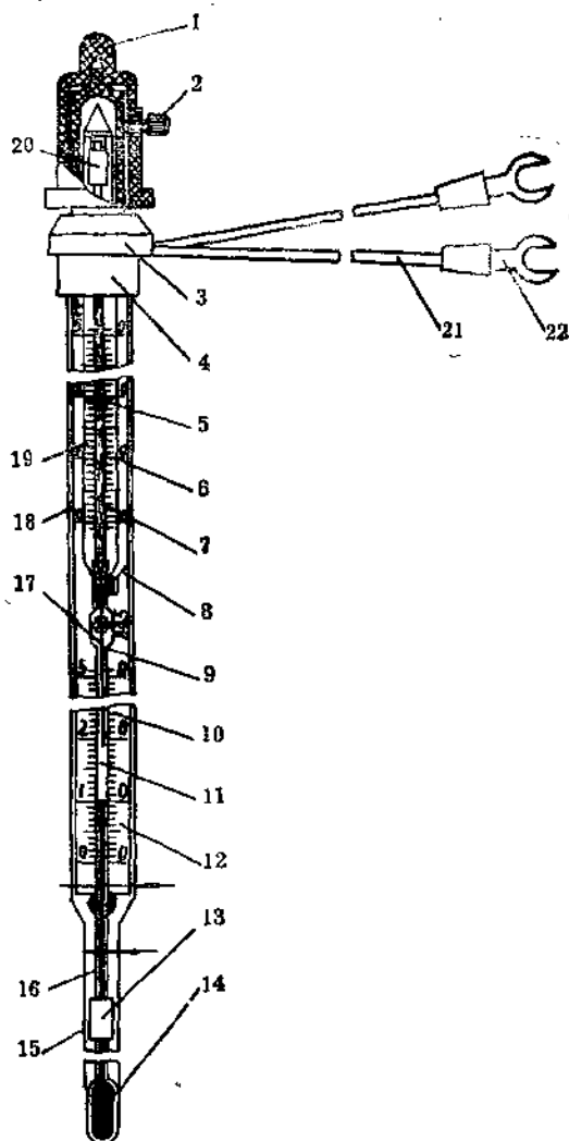
图1 可调式温度计
