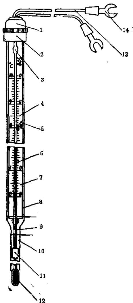
图2 固定式温度计
