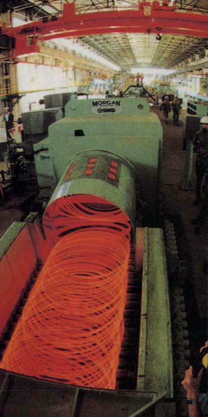
马钢高速线材厂(十七冶机电公司承建安装)
