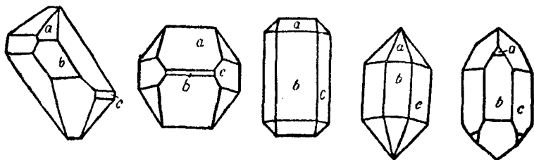
图 1-2. 石英结晶外形。
