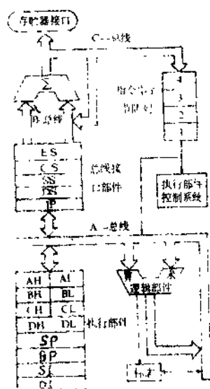
图3—1 8088的框图
