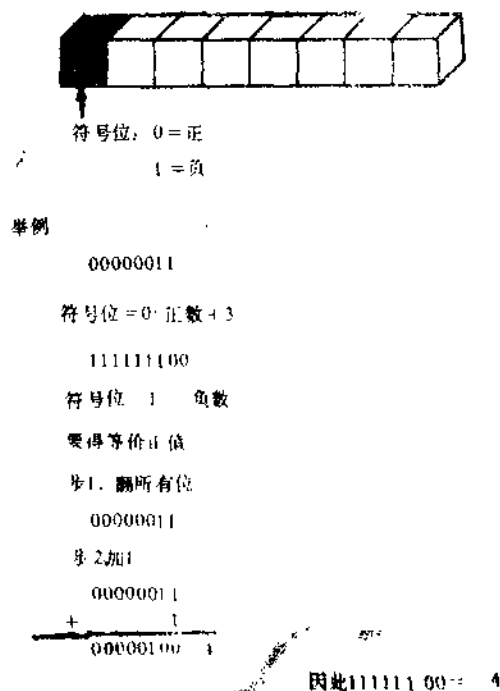
图 2—9 二进制补码数
