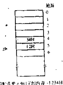
存储器单元4的内容=1234H
