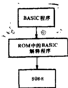
图1-1 解释执行
