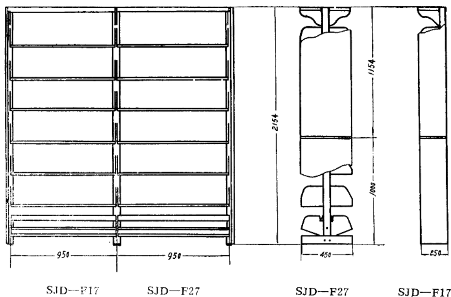
侧 视 图
