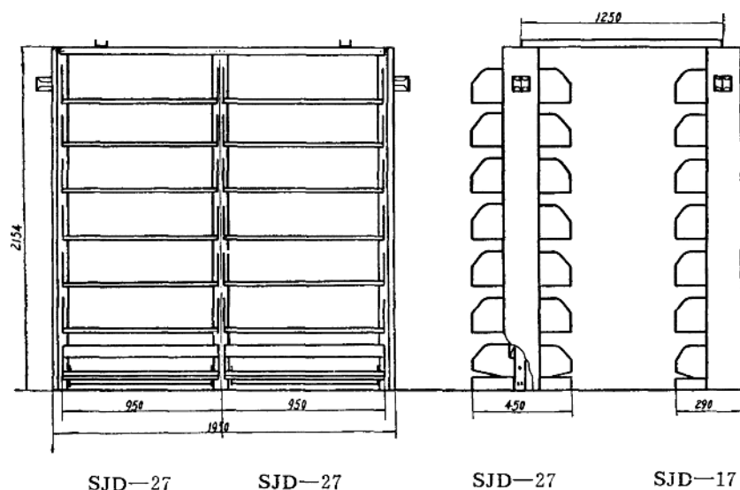
SJD单柱书架技术参数
