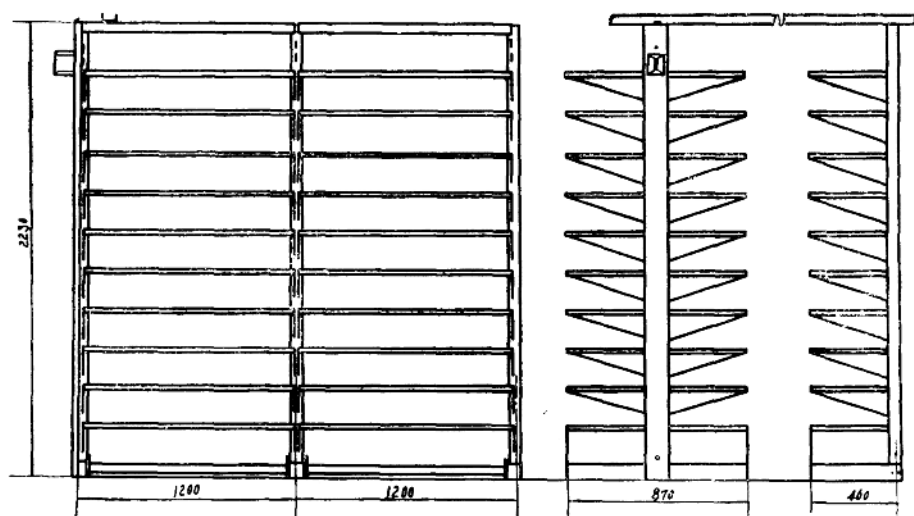
正 视 图
