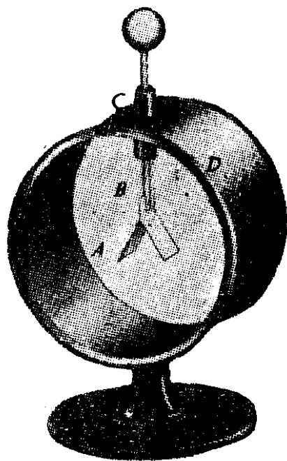
图 24-1 箔验电器。
