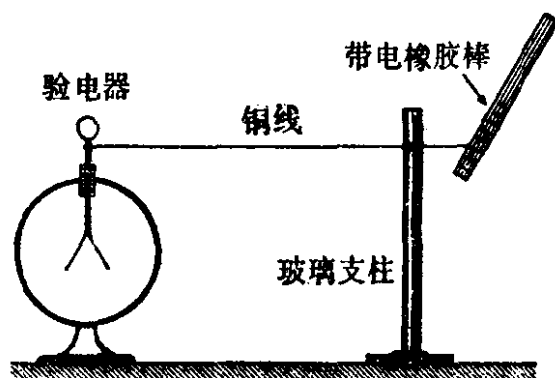
图 24-2 铜是导体。
