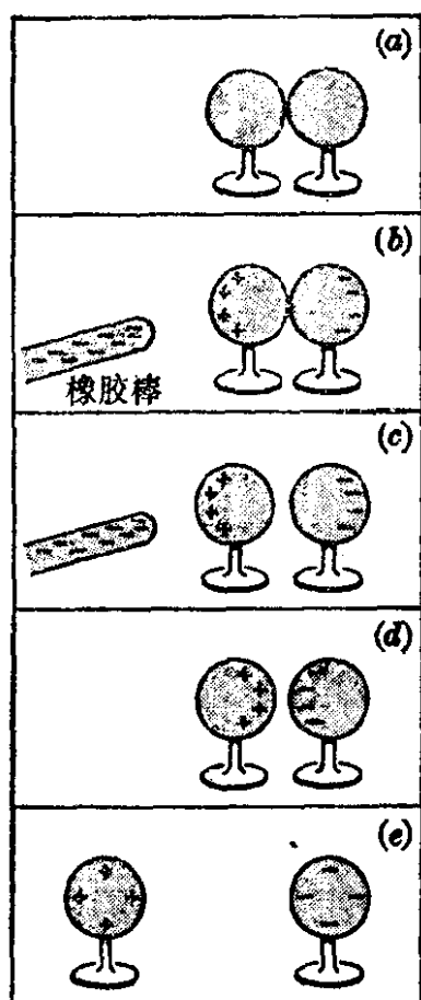
图 24-3 感应起电使两个金属球带异号电。
