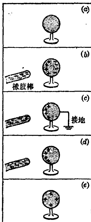
图 24-4 感应起电使单个金属球带电。
