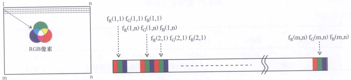
图2-11 按各波段的同一像素点依次存储
