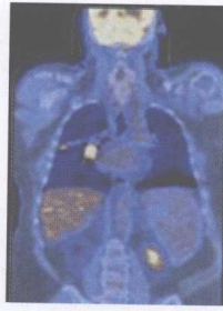
图8-8 PET-CT成像
