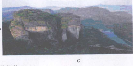
图2-22 图像的衔接
