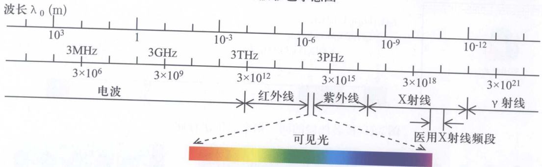
图3-1 电磁波谱图
