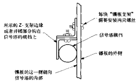
图 1-10 天线塔梯的横挡上安装屏蔽装置。
