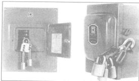
图1-6 在爬天线塔之前,应将天线开关及电源开关切断,并在盒上加锁并加挂警示牌“严禁合闸”。
