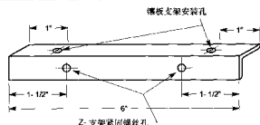
图 1-8 Z-支架元件片。
