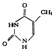
胸腺嘧啶
