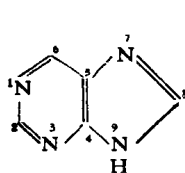
嘌呤
