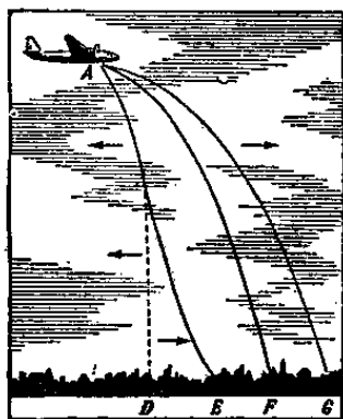
图3. 飞机上投下的炸弹所走的路径： AF ，在没有风的天气里； AG ，在顺风的时候； AD ，在逆风的时候； AE ，在上面逆风、下面顺风的时候。
