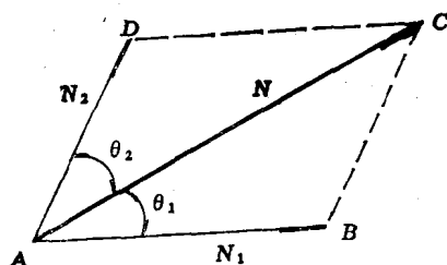
图1-1 力的平行四边形法则
