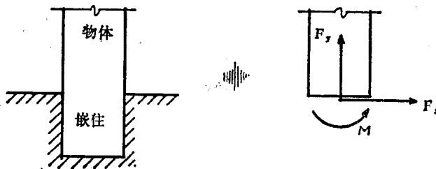
图1-6 固定端约束
