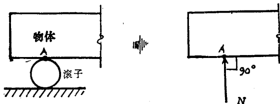
图1-4 滚轴约束
