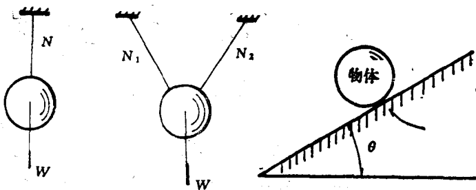
图1-2 柔性约束
