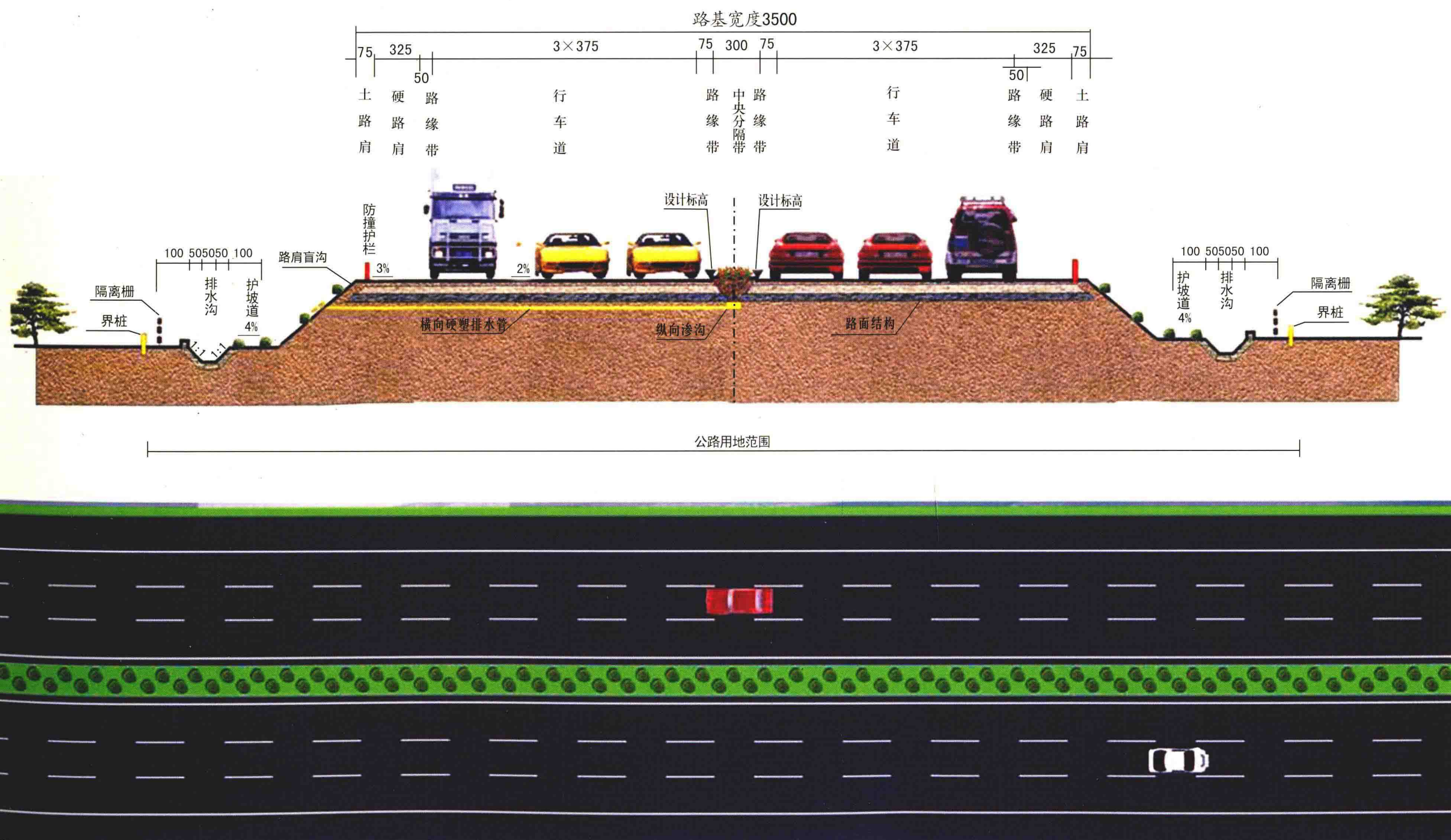
路基标准横断面图
