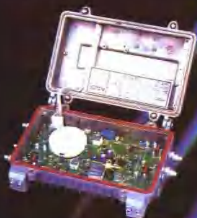
野外型调幅激光接收机
