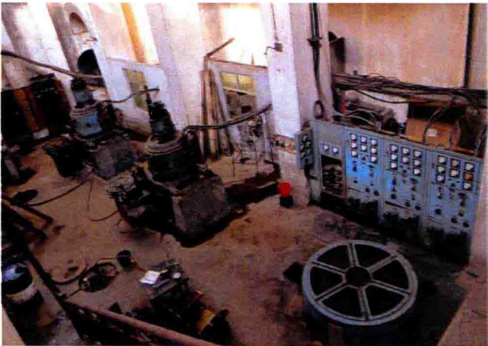
段家塘电站发电机组室
