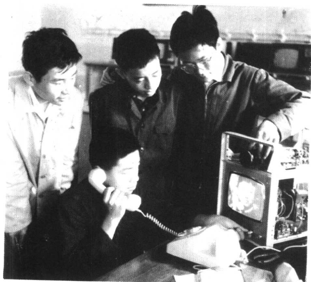
北京市少年宫无线电小组试制成功“可视电话” 获全国第二次青少年科技作品金牌
