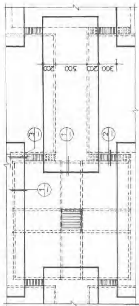
吊顶局部布置图
