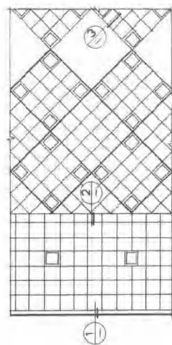
影剧院前厅吊顶仰视图局部
