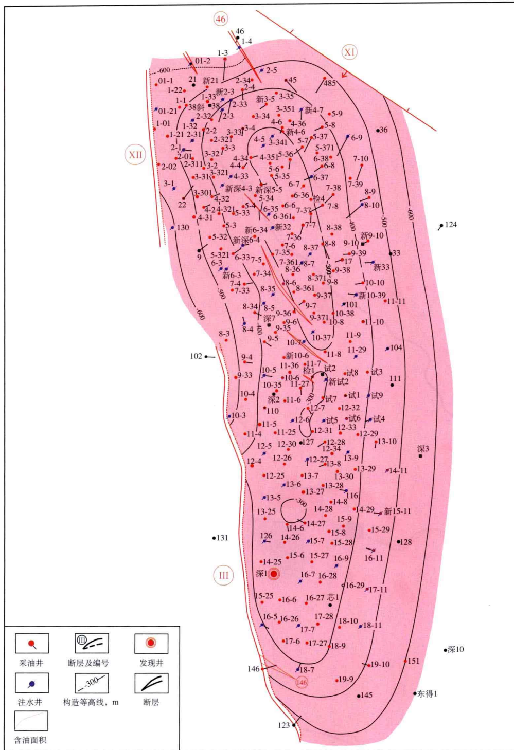
尕斯库勒油田 E 3 1 油藏构造井位图 (青海油田分公司勘探开发研究院绘制, 2005 年)
