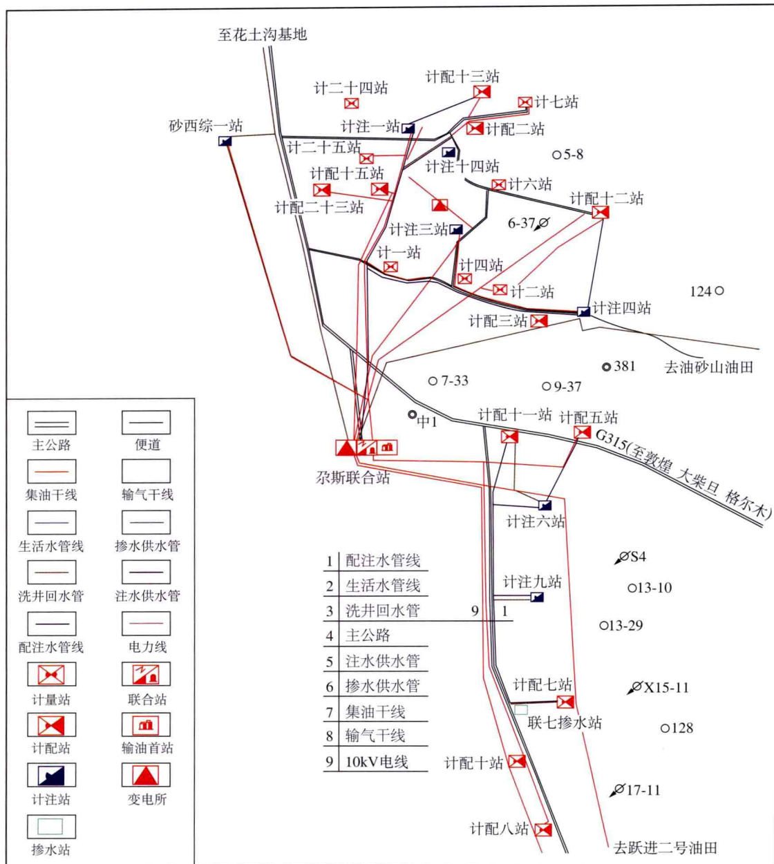
青海杂斯库勒油田地面建设总图 (CPE 青海分公司绘制, 2005 年)
