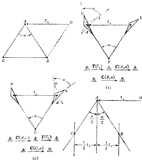
图 1-2 平移与旋转的归并定理
