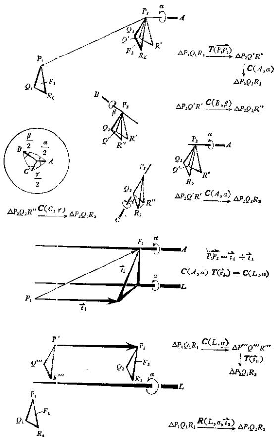
图 1-5 第一类重合操作和有关定理
