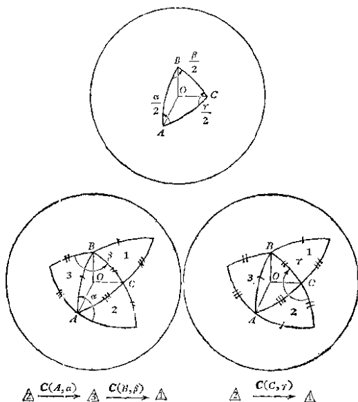
图 1-1 两个旋转的归并定理(Euler 定理)
