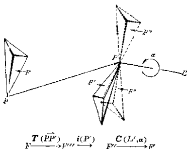
图 1-6 第二类重合操作和有关定理
