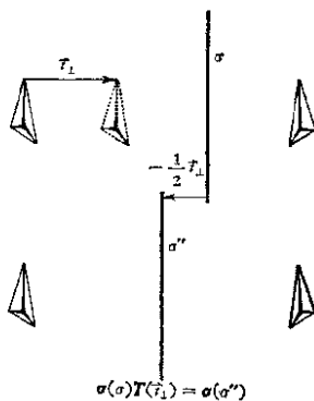
图 1-3 平移与反映的归并定理
