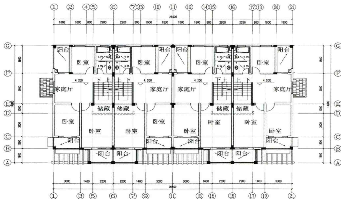
二层平面图
