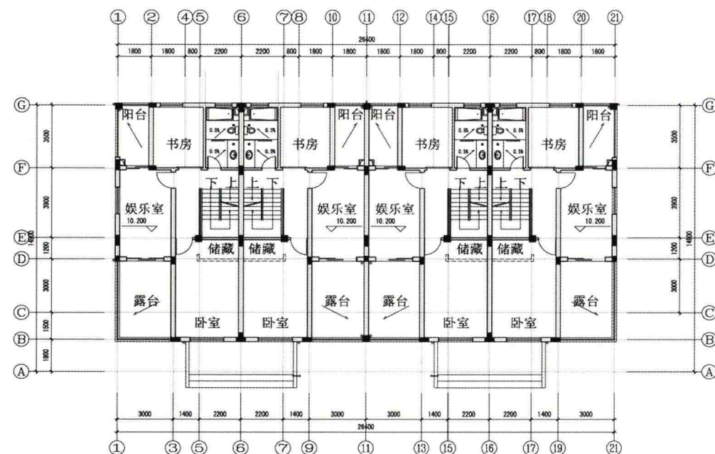
四层平面图
