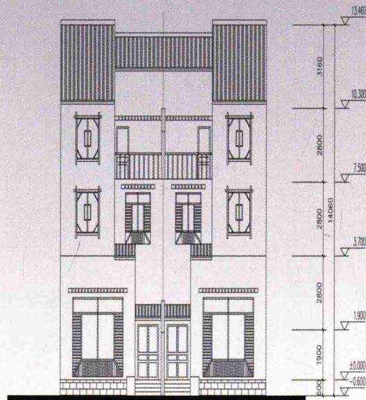
双联南立面图
