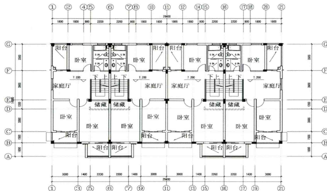
三层平面图
