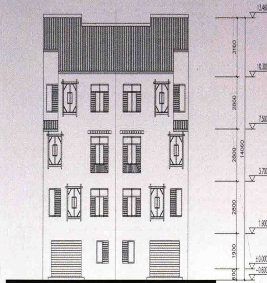
双联北立面图
