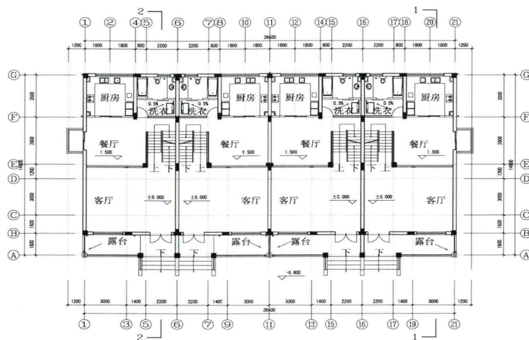
一层平面图
