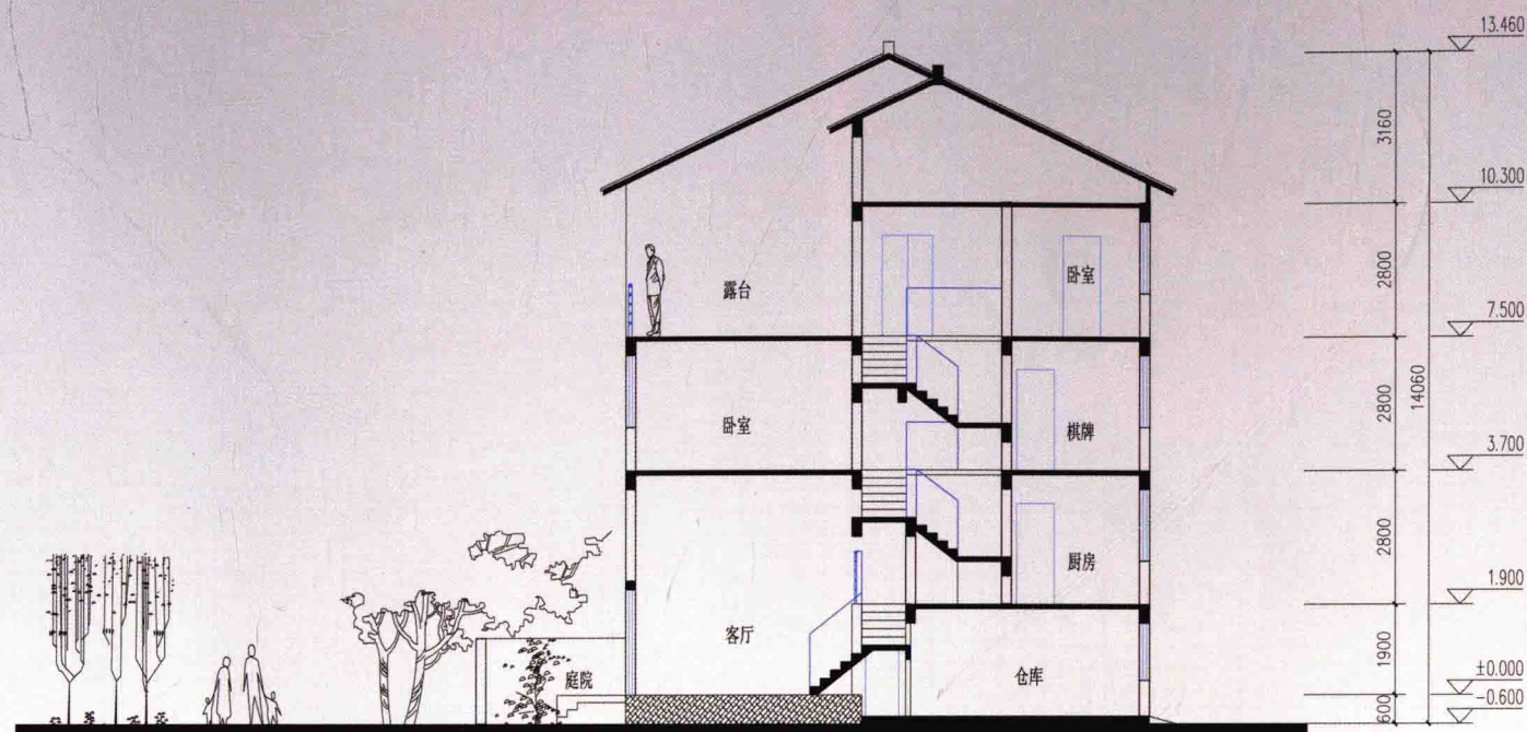
1-1 剖面图
