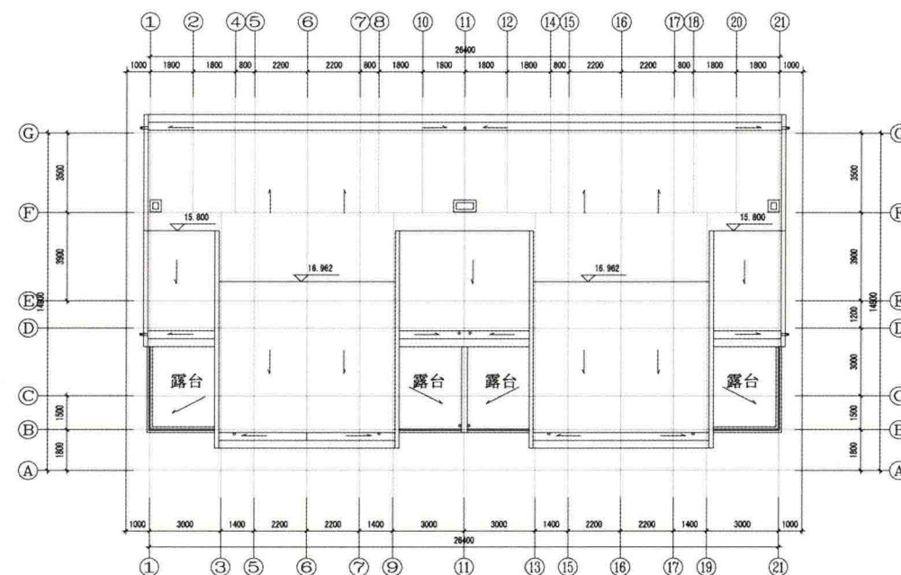
屋顶平面图
