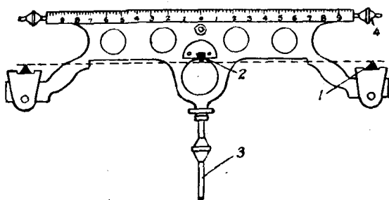
圖 2. 天平梁及刀口的位置: 1—天平梁两端的刀口; 2—中间的刀口; 3—指针; 4—调节零点的螺丝。
