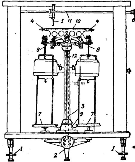
圖 6. 空气阻尼式天平。
