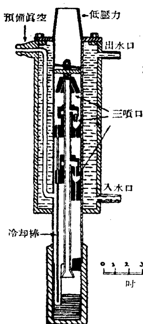
圖10 給德抽氣機
