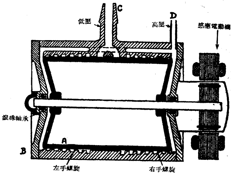
圖 7 好來維克分子抽氣機
