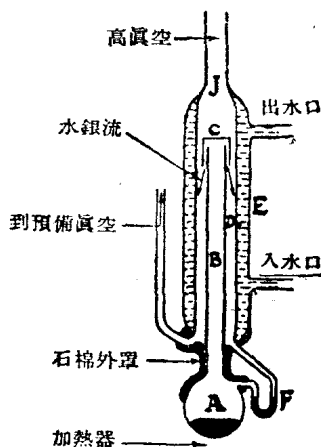
圖 8 水銀擴散抽氣機
