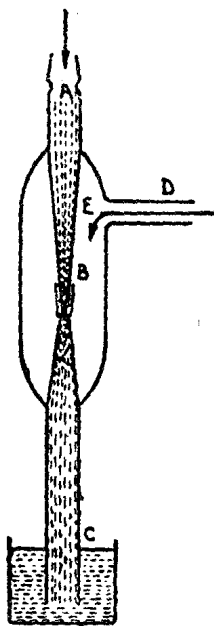
圖 1 水流抽氣機
