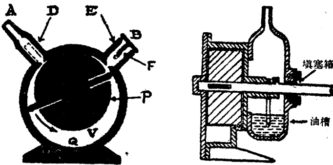
圖 2 給德機械式“輔助”抽氣機
