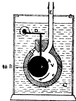
圖 5 信扣海維克“輔助”抽氣機
