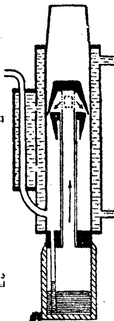
圖11 喀義抽氣機
