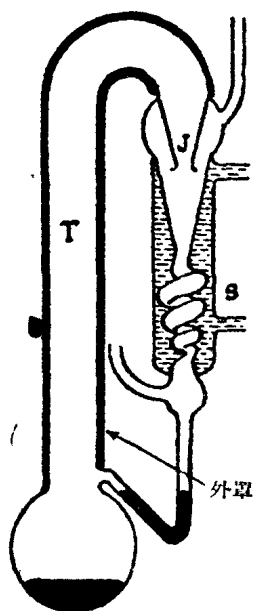
圖9 凡摩而抽氣機
