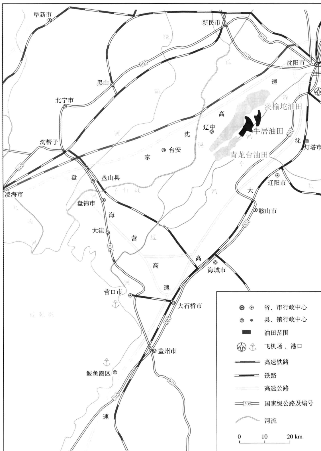
牛居油田地理位置图 (辽河油田茨榆坨采油厂编制, 2009 年)
