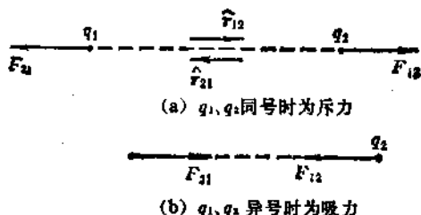
图 1-5 用库仑定律的矢量形式判断两个点电荷间静电力的方向。
