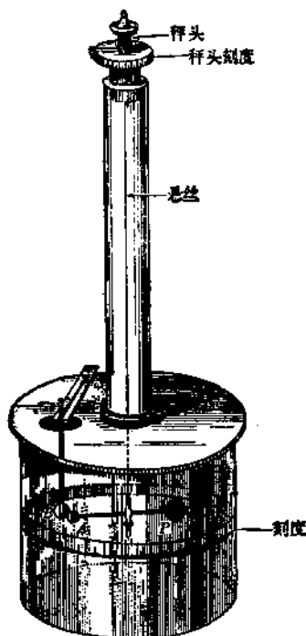
图 1-2 库仑扭秤
