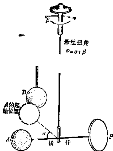
图 1-3 银丝扭角的计算
