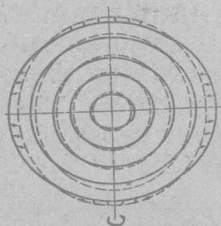
图 1-3 地球由圓形趋向橢球的变化示意图
