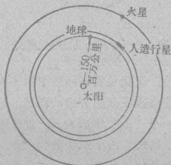
图 1-2 人造行星运行示意图
