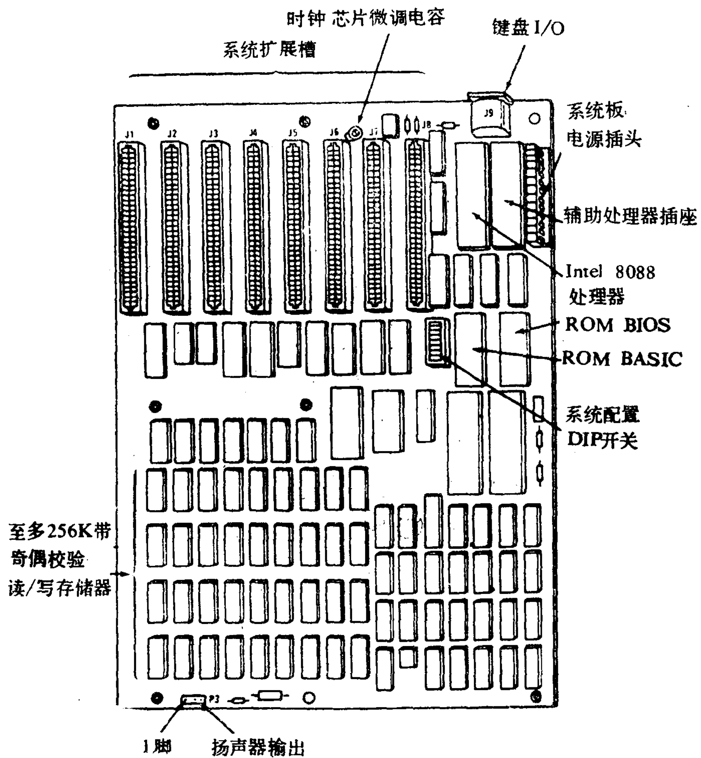
系统板元件图
