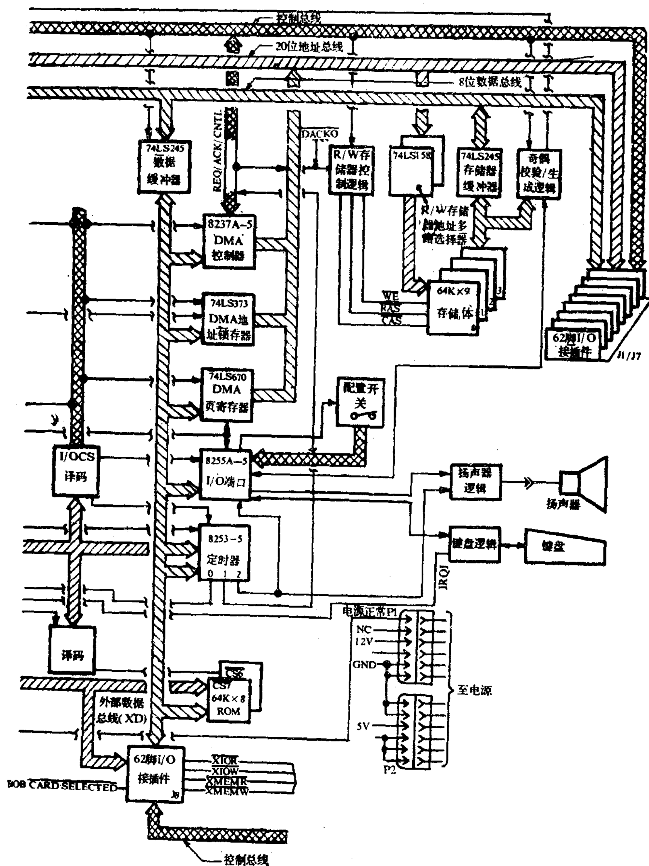
系统板数据流 (2 之 2)
