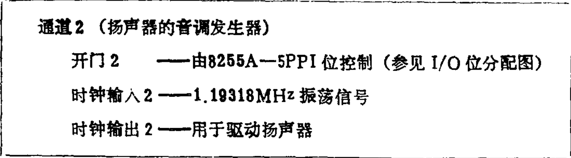
扬声器音调发生器
