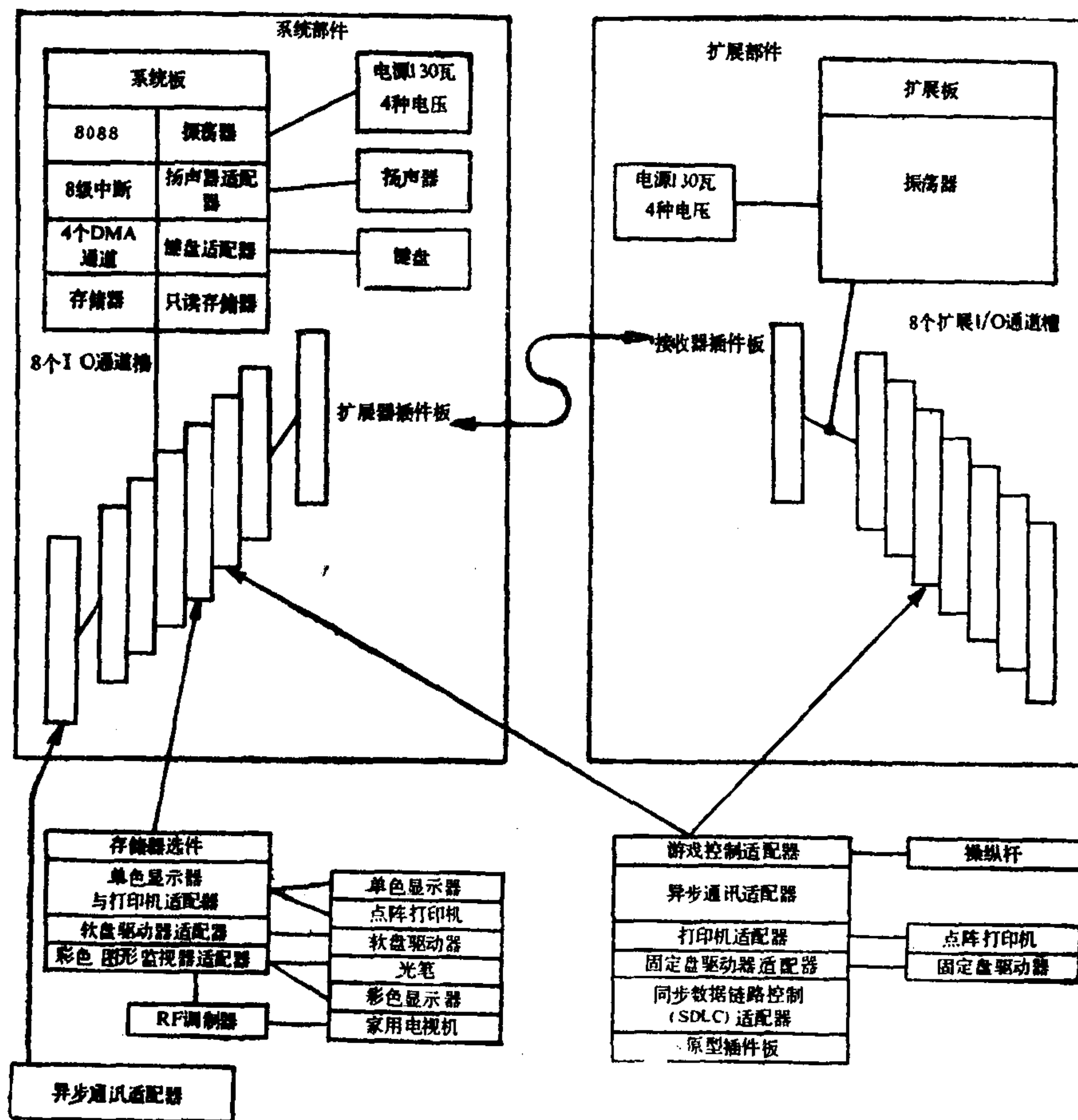
系统框图
