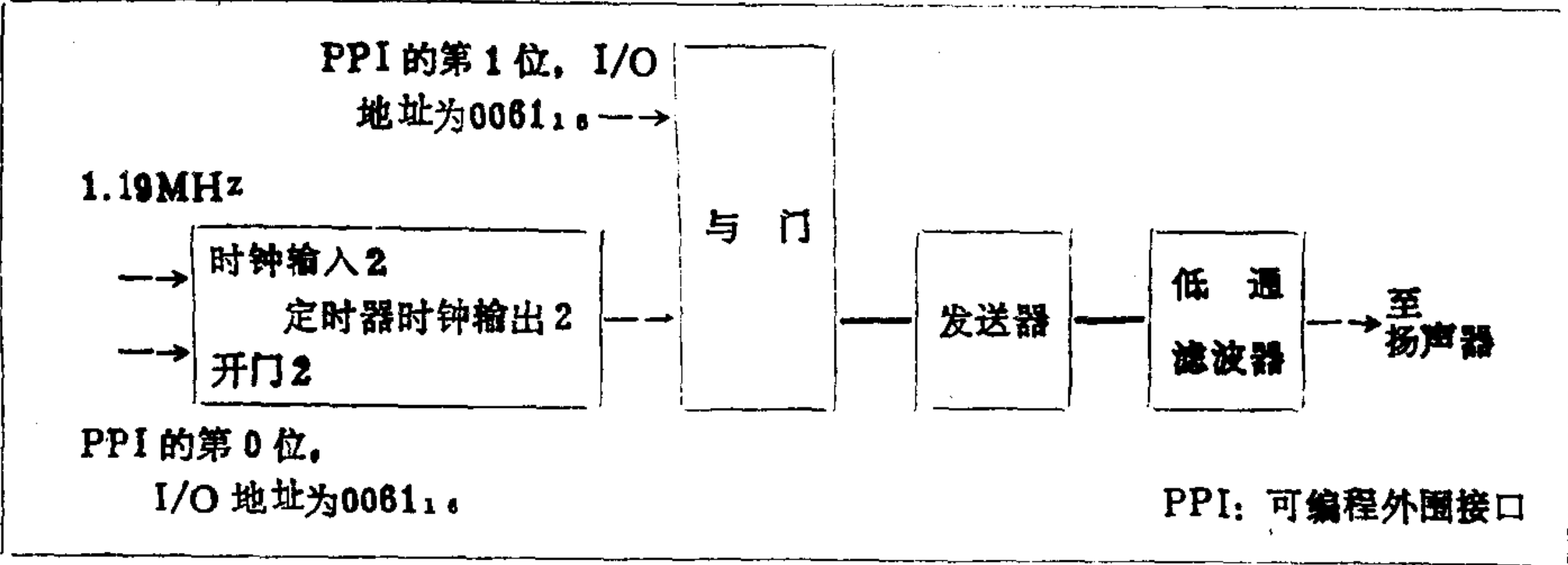
扬声器驱动系统框图
