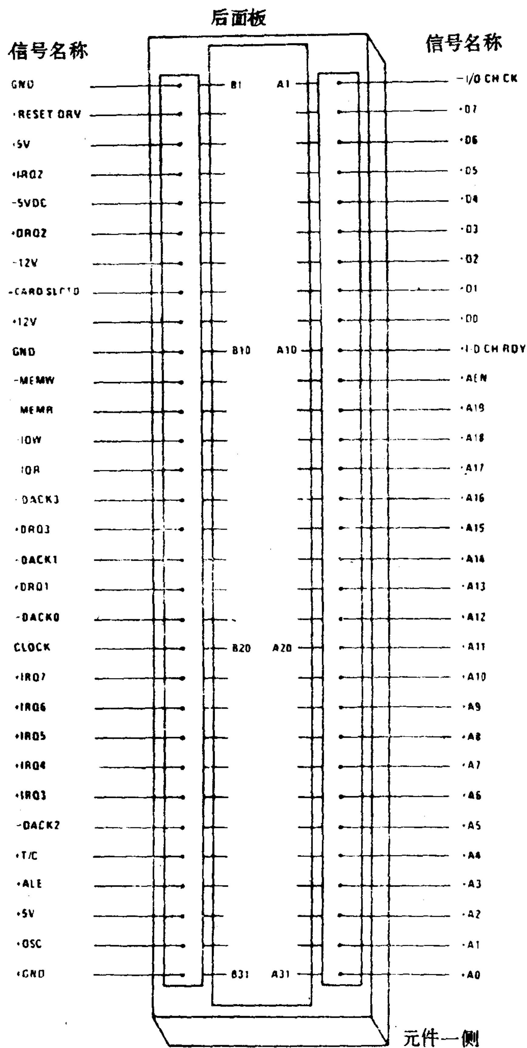
I/O 通道图
