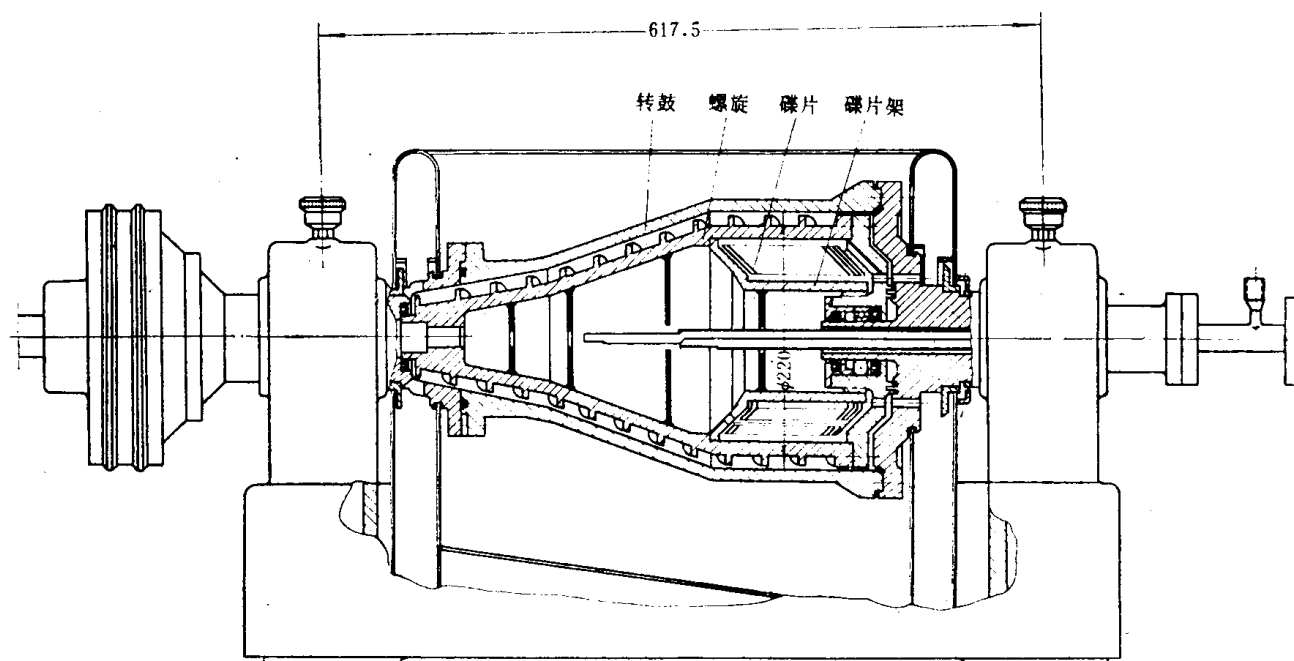
图78-1-14 卧式螺旋碟片复合式离心机
