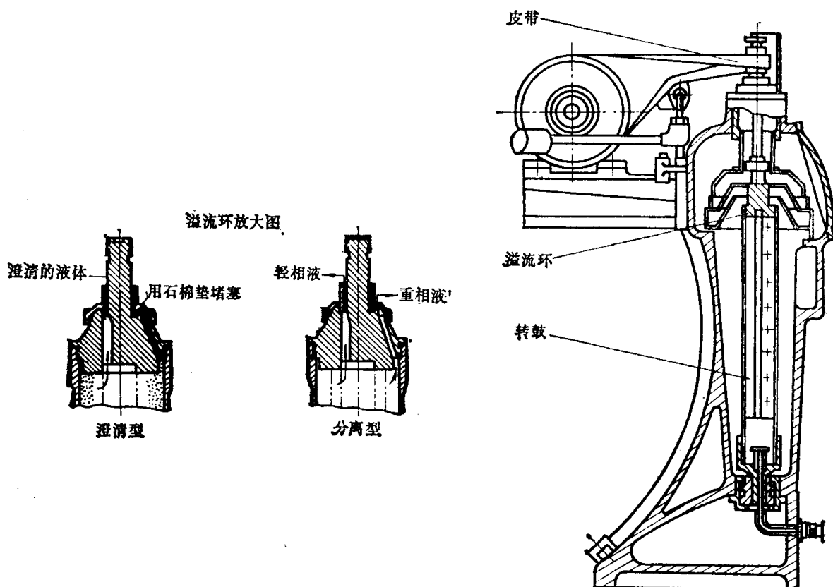
图78·1-9 管式分离机
