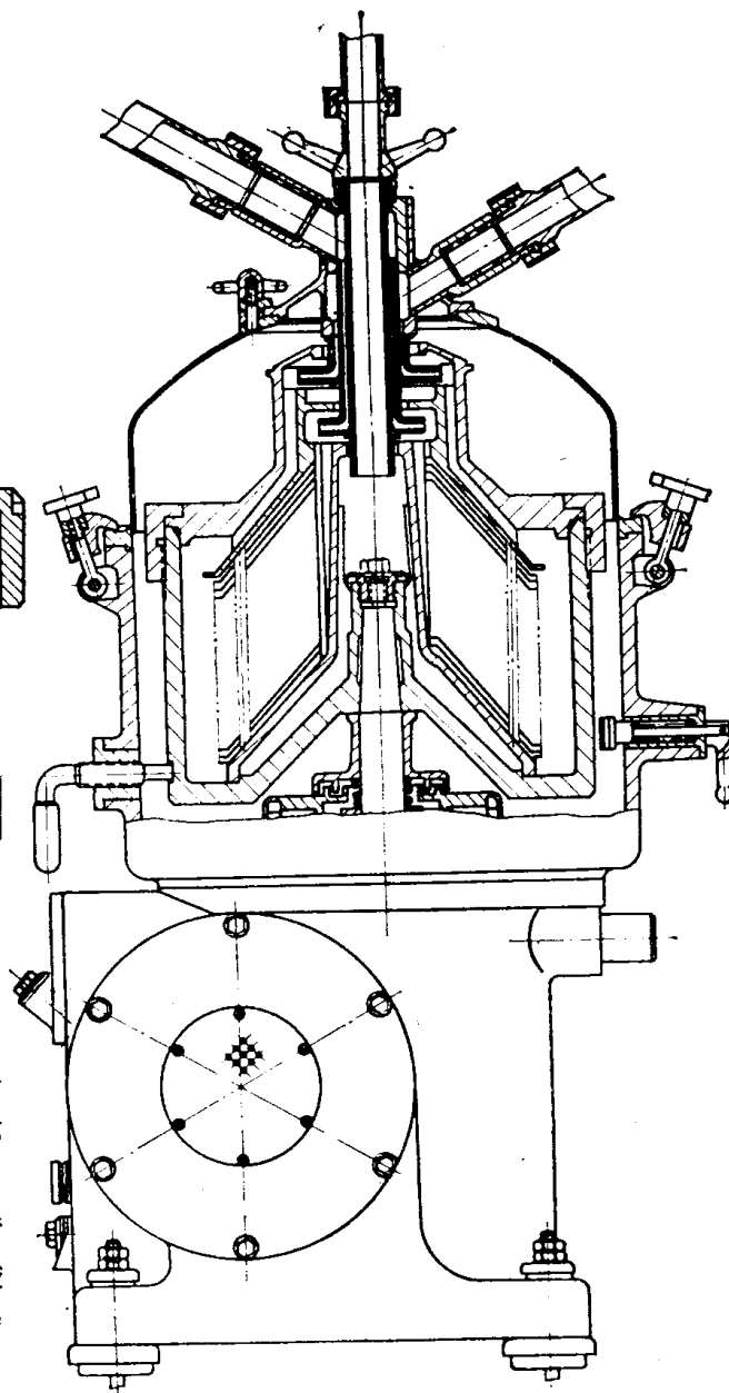
图78·1-11 碟式人工排渣分离机
