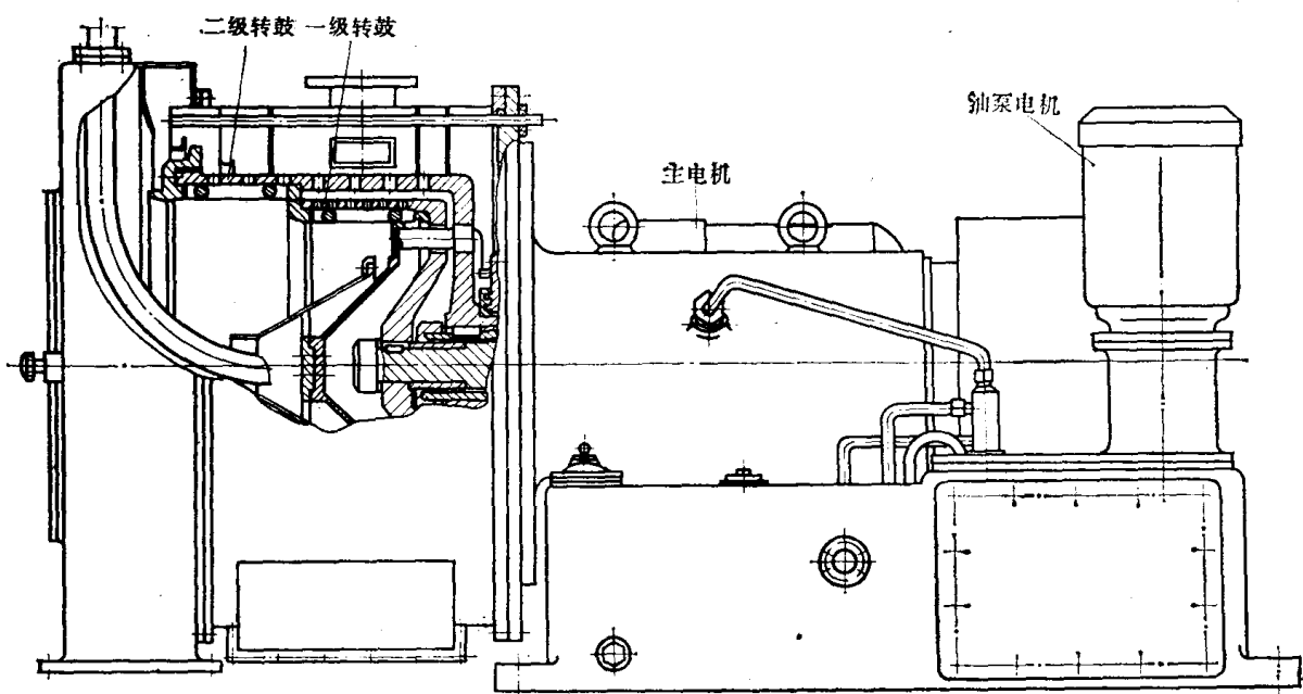
图78·1-4 卧式双级活塞推料离心机
