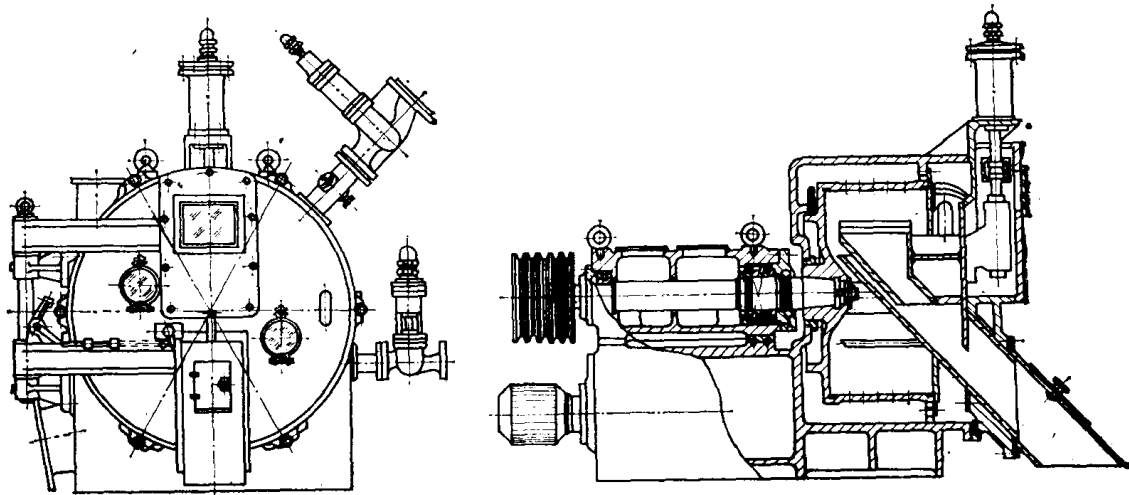
图78·1-3 卧式刮刀卸料离心机
