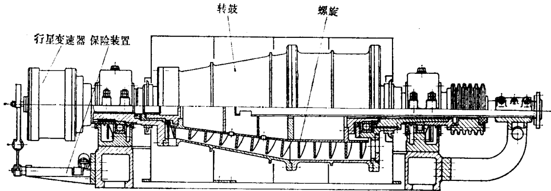
图78·1-8 卧式螺旋卸料沉降离心机
