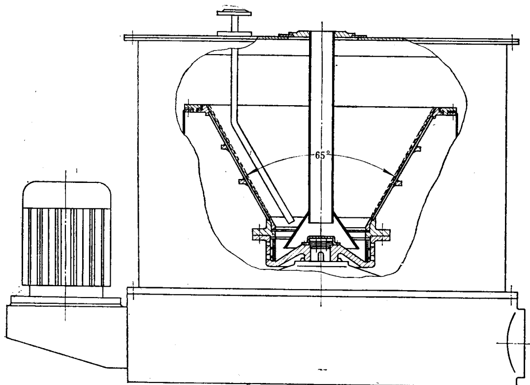
图78·1-5 立式离心力卸料离心机
