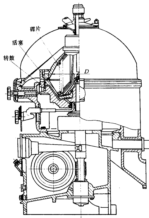
图78-1-13 碟式活塞排渣分离机
