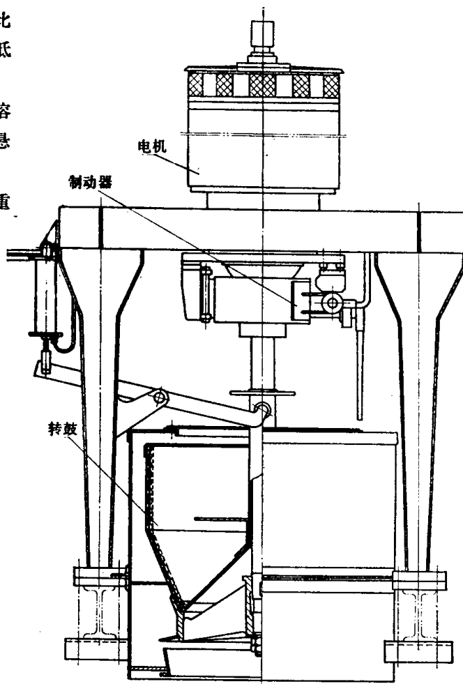
图78-1-2 上悬式重力卸料离心机
