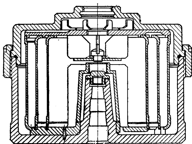
图78·1-10 室式分离机
