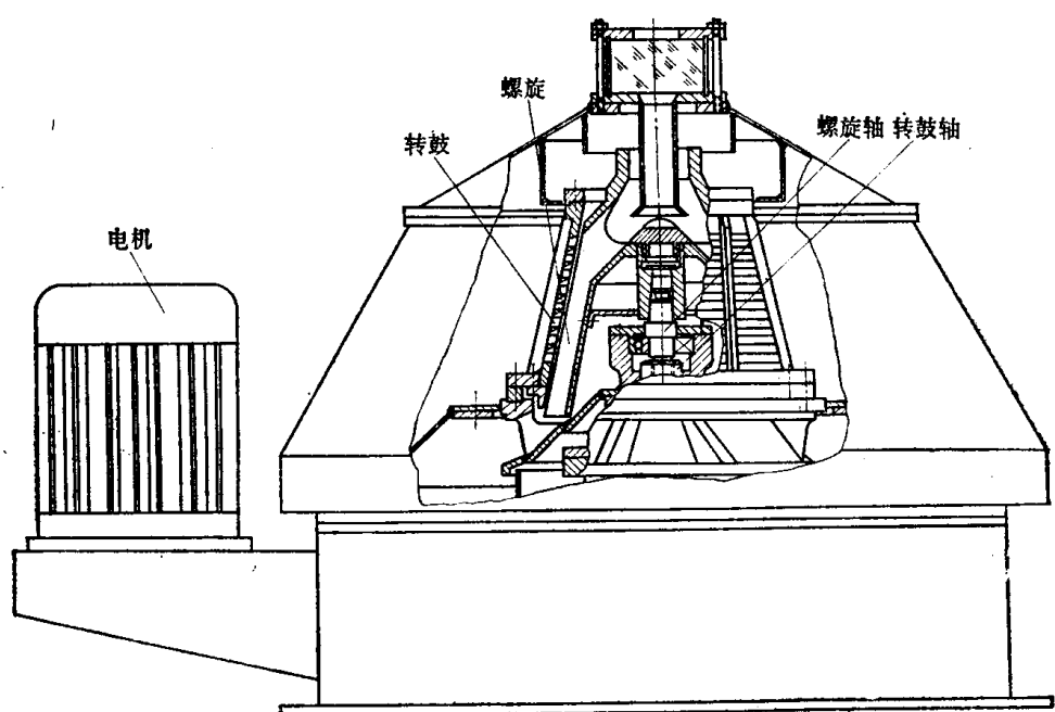
图78-1-7 立式螺旋卸料过滤离心机
