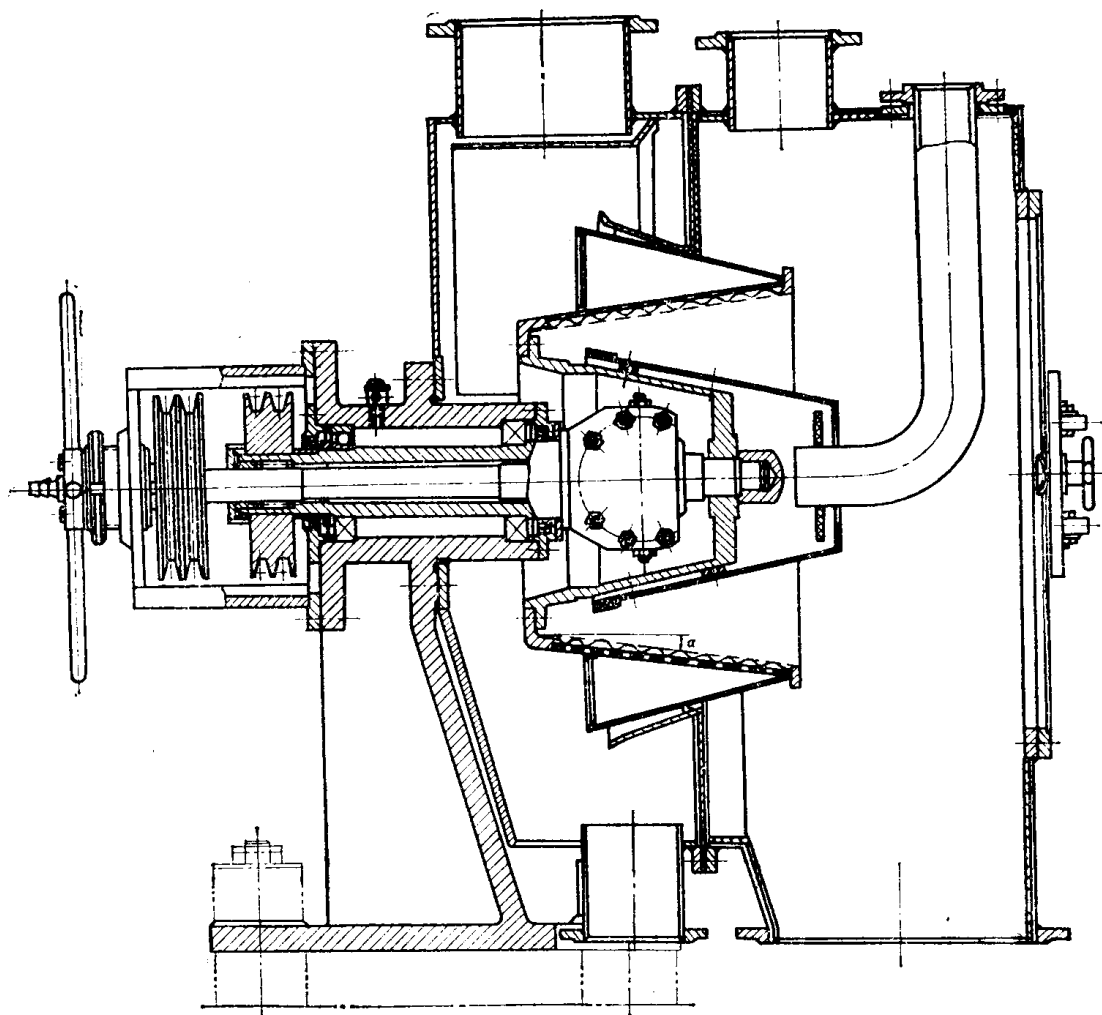
图78-1-6 卧式进动卸料离心机
