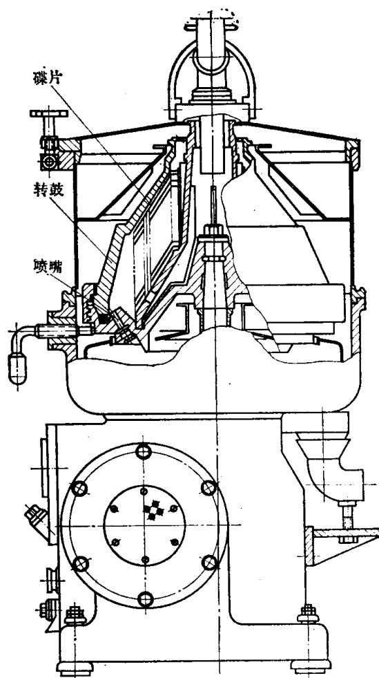
图78-1-12 碟式喷嘴排渣分离机
