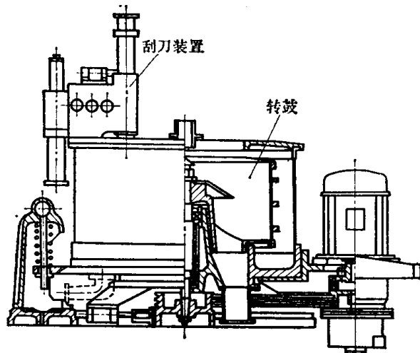
图78-1-1 三足式下部自动卸料离心机
