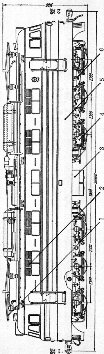
图 3 H60型电力机车的主要尺寸：
