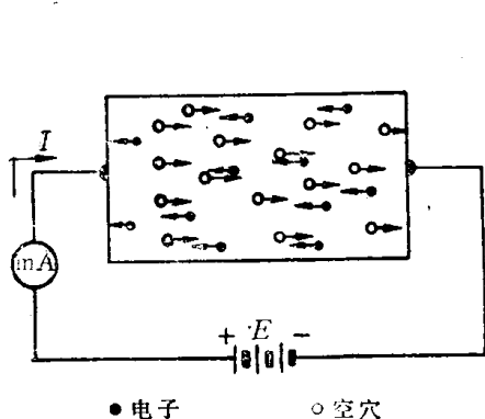
图1-1-5 半导体中的漂移电流
