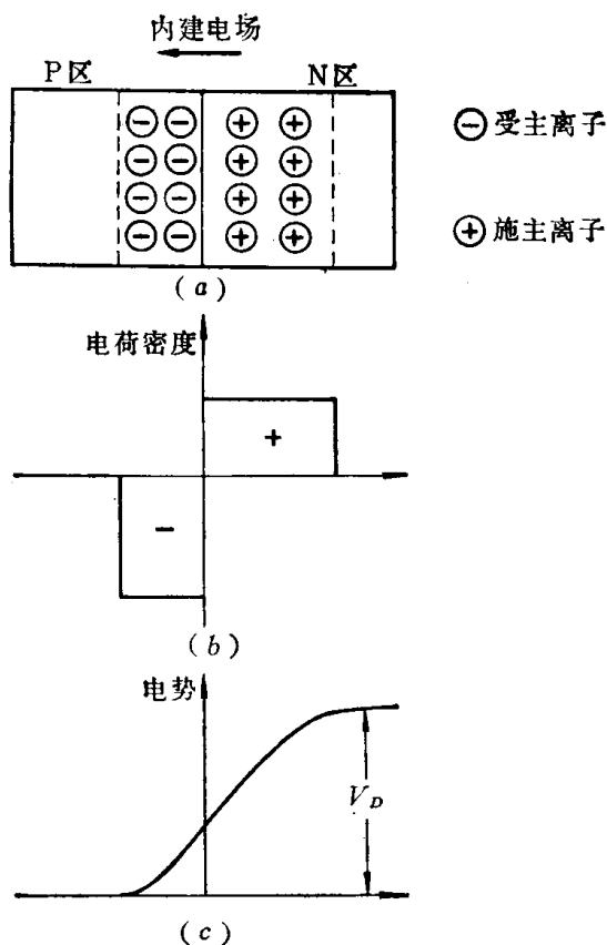
图1-2-1 PN结势垒区
