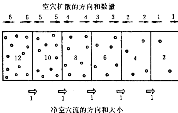
图1-1-6 说明扩散电流的一维模型
