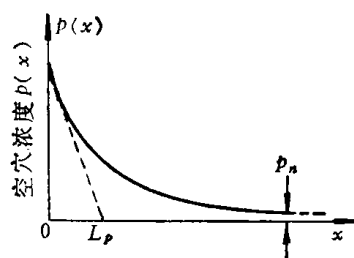
图1-2-3 在正向电压作用下N区空穴的分布
