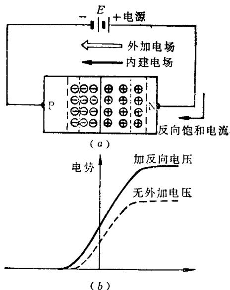
图1-2-4 外加反向电压的PN结
