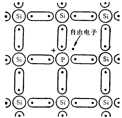
图1-1-3 N型半导体结构示意图
