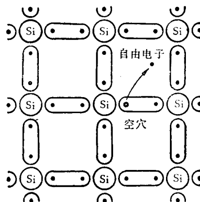
图1-1-2 一个共价键断裂，产生一个电子空穴对
