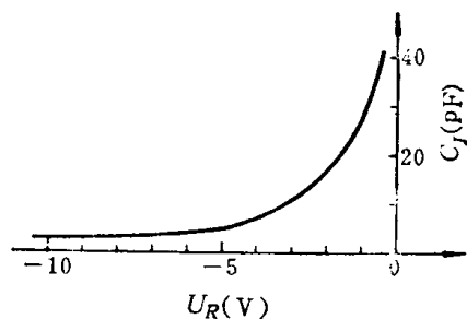
图1-2-5 B11型变容二极管 C_j - U_R 特性
