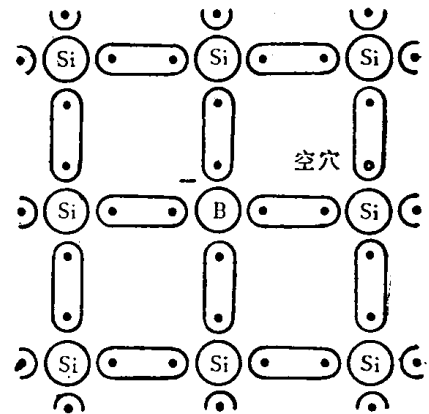
图1-1-4 P型半导体的原子结构示意图
