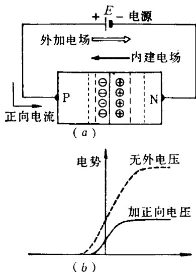
图1-2-2 外加正向电压的PN结
