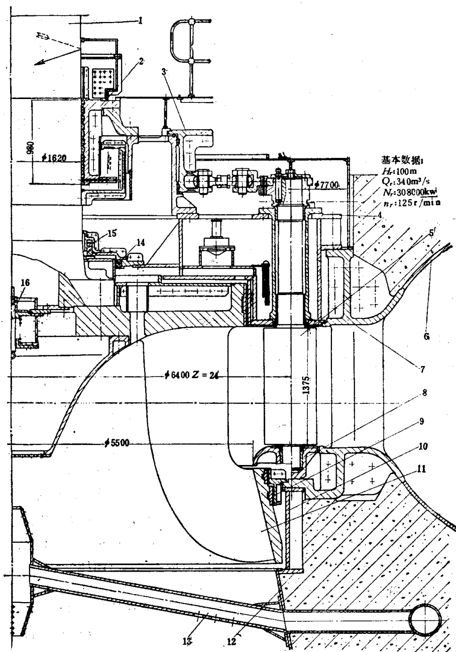
图75·1-3 300×10 3 kW混流式水轮机剖面图
