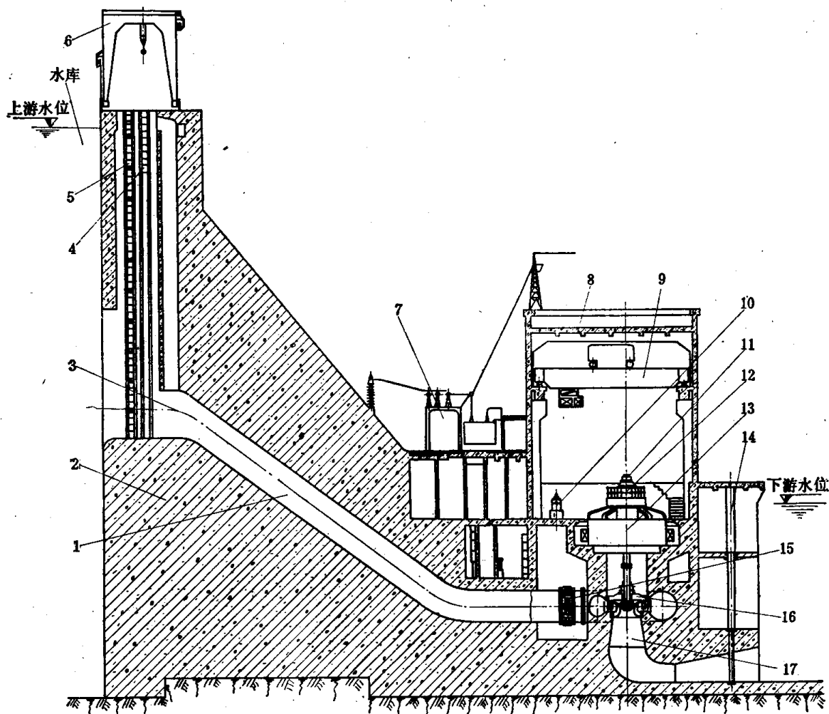
图 75·1-1 坝后式水电站剖面图
