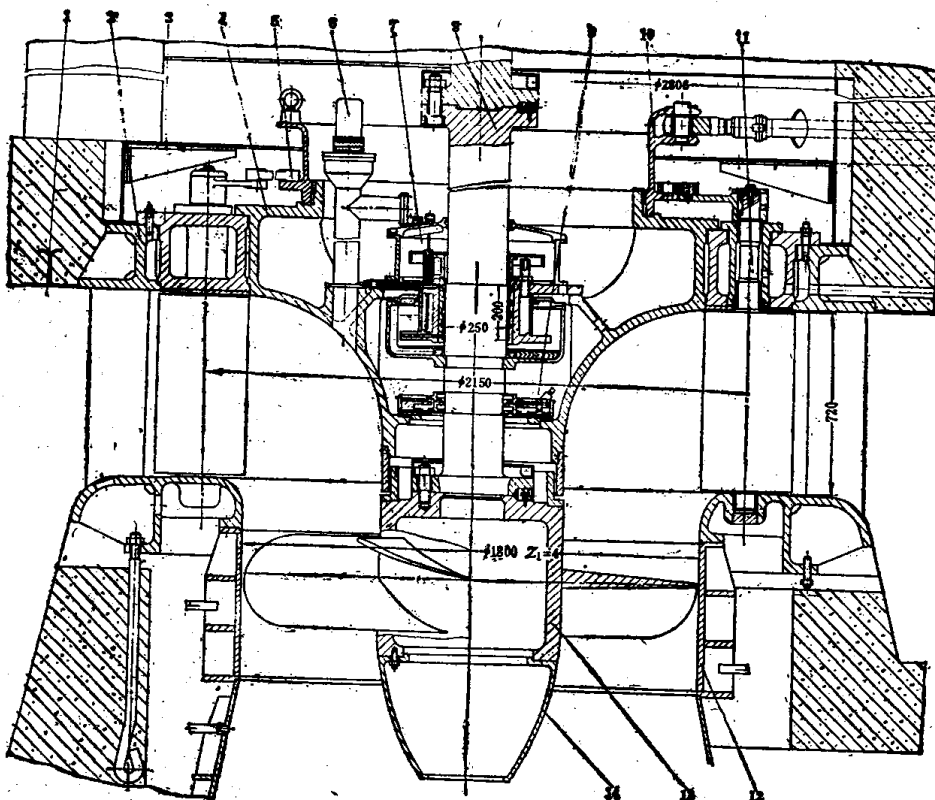
图75-1-8 轴流定桨式水轮机剖面图
