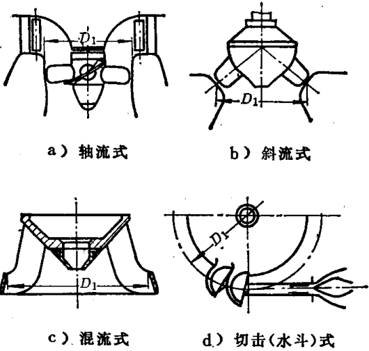
图75-1-2 转轮标称直径
