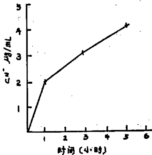
图2 铁氰复盐分解与光照的关系。
