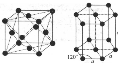
图 1-5 晶体结构图形
