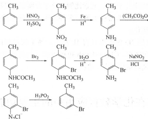
图 1-2 甲苯制间溴甲苯反应过程示意图
