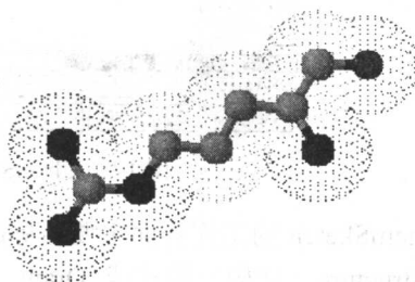
图 1-7 具有电子云的 3D 分子结构
