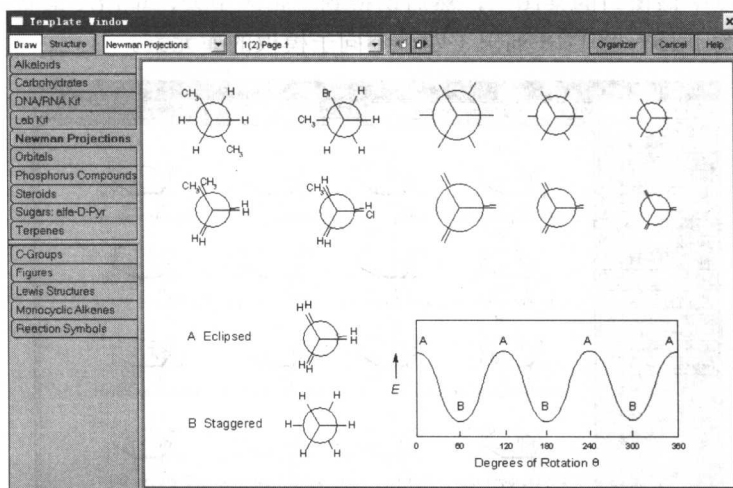
图 1-18 纽曼结构式子模板
