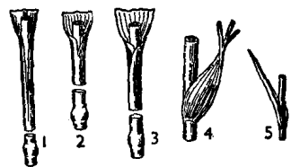
叶鞘 1.敞鞘 2.闭鞘 3.卷鞘 4.腋鞘 5.狭叶鞘
