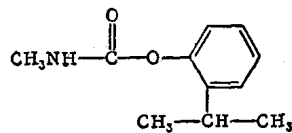
叶蝉散结构式
