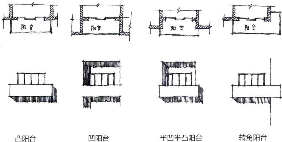
图2-5 阳台的形式
