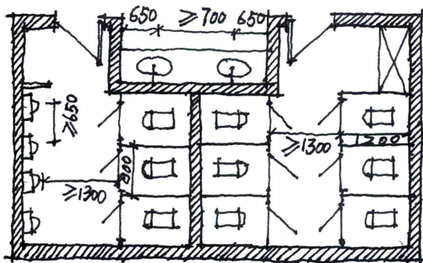
图2-6 卫生间的形式
