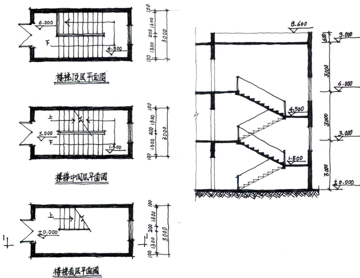
图2-2 基本楼梯的平面图和剖面图
