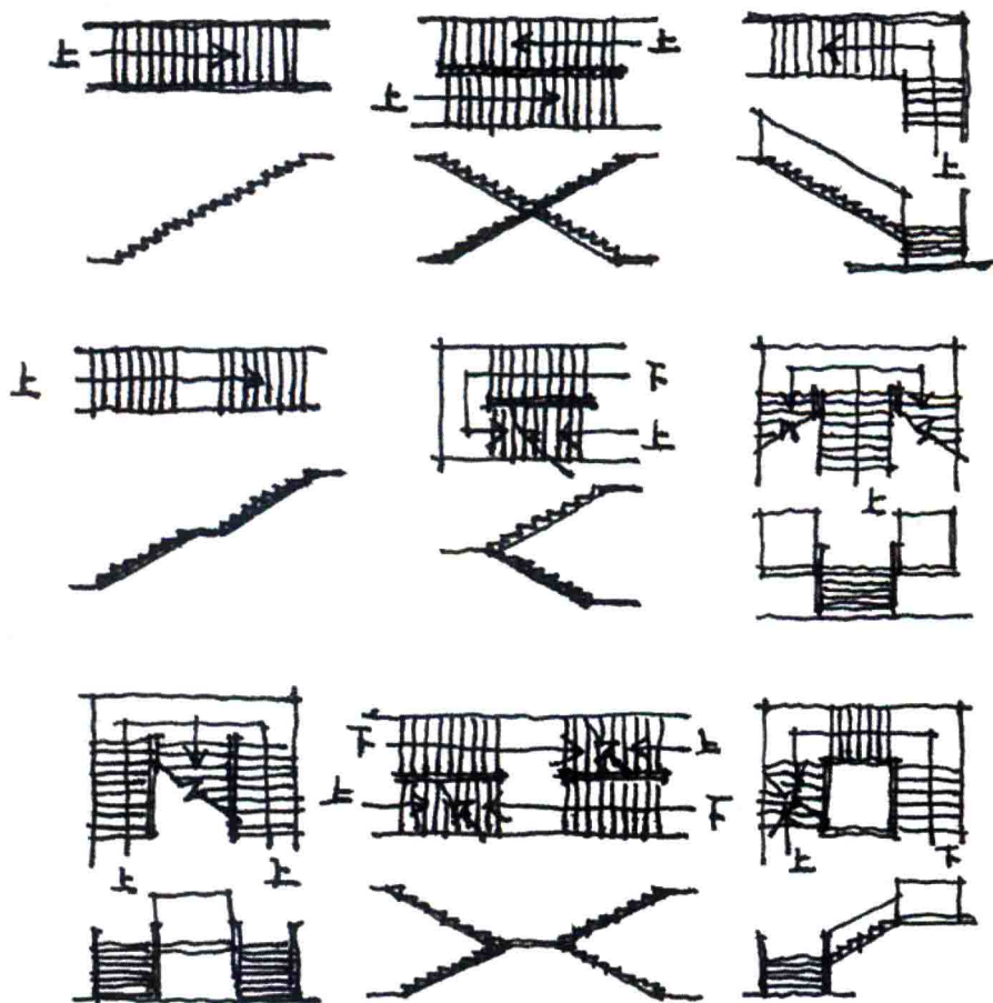
图2-4 楼梯的各种形式
