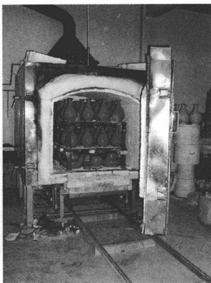
图1-2 现代煤气窑
