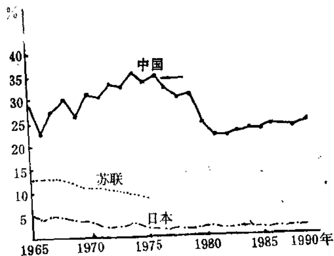
图3 铸造铁占生铁总产量的比重 (铸铁比)
