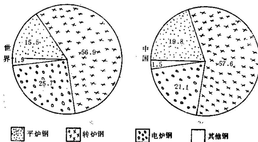
图4 按炼钢方法划分钢产量构成比
