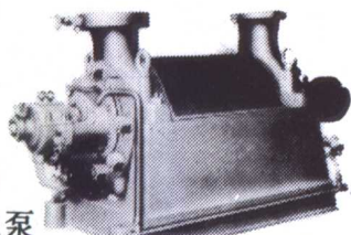
GZ270~150型水力采煤泵 270米 3 /时 750~1350米 2980转/分
