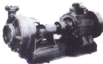
6J35型胶粒悬浮液泵 105~160米 3 /时 15~35米 970~1480转/分
