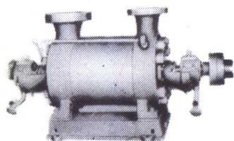
GZ270~150型水力采煤泵 270米 3 /时 750~1350米 2980转/分
