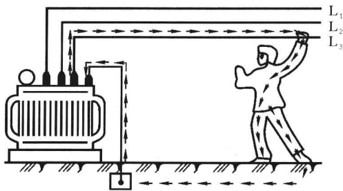
图 1-1-2 中性点直接接地系统的单相触电
