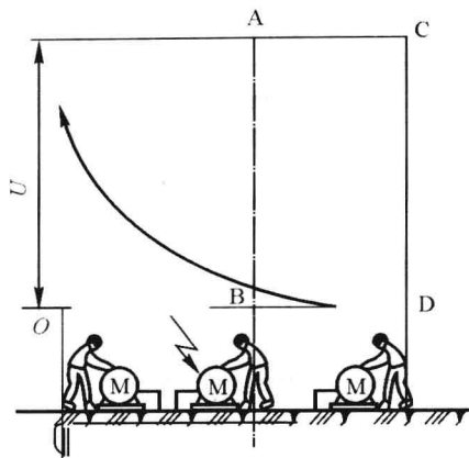
图 1-1-7 接触电压触电
