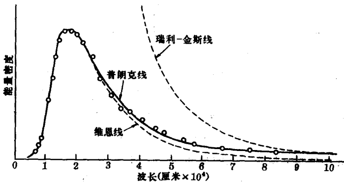
图2 黑体辐射能量分布曲线
