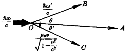
图 3 康普顿散射
