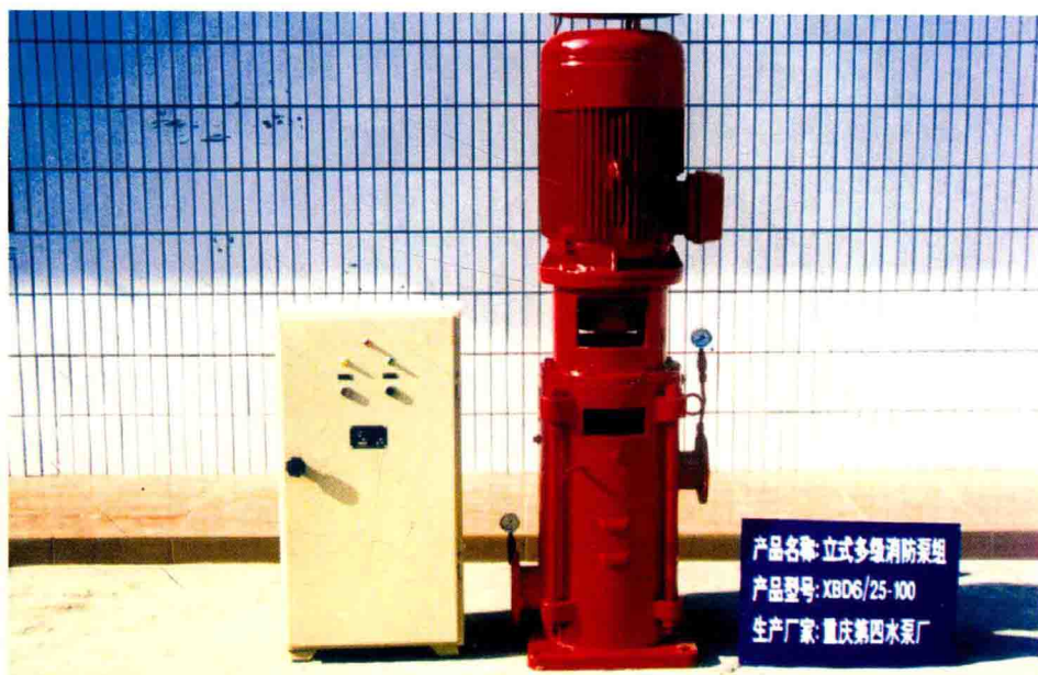
▼ XBD 立式多级消防泵组
