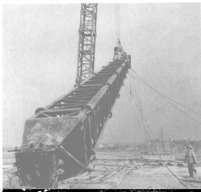
竖塔架，采用桅式塔架，一省钢材二省时间，施工也较方便。
