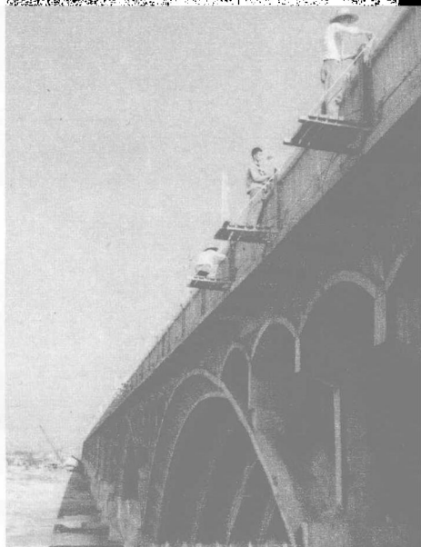
水刷石栏杆柱。
